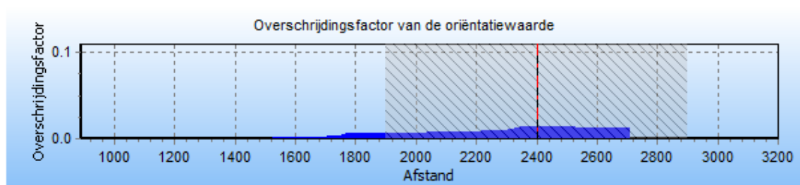
4.7 Figuur 4.7 Groepsrisico screening voor 6344_leiding-N-576-02-deel-1 van N.V. Nederlandse Gasunie
