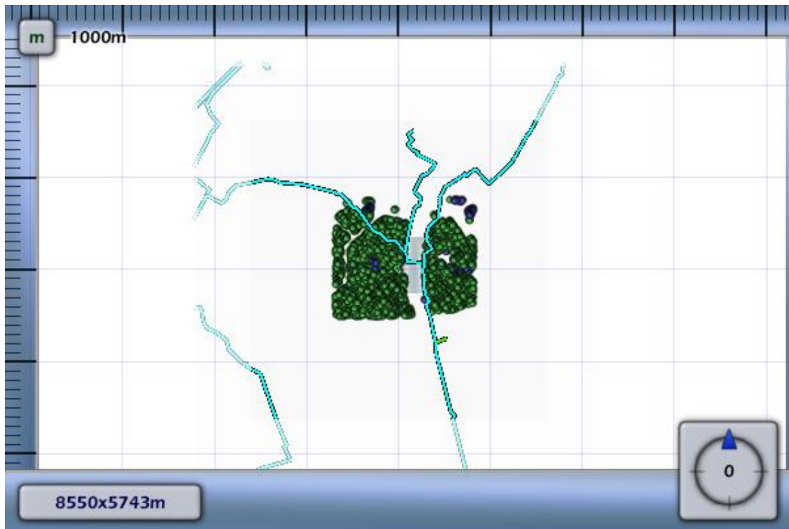
4.11 Figuur 4.11 Groepsrisico screening voor 6344_leiding-N-576-70-deel-1 van N.V. Nederlandse Gasunie
