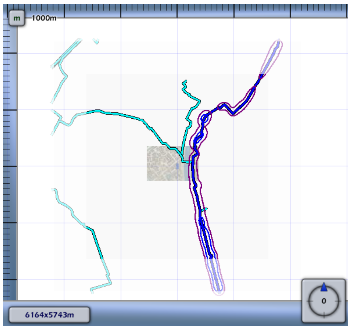
3.8 Figuur 3.8 Plaatsgebonden risico voor 6344_leiding-N-576-67-deel-1 van N.V. Nederlandse Gasunie
