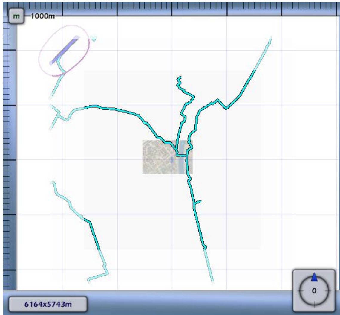
3.2 Figuur 3.2 Plaatsgebonden risico voor 6344_leiding-A-533-deel-1 van N.V. Nederlandse Gasunie
