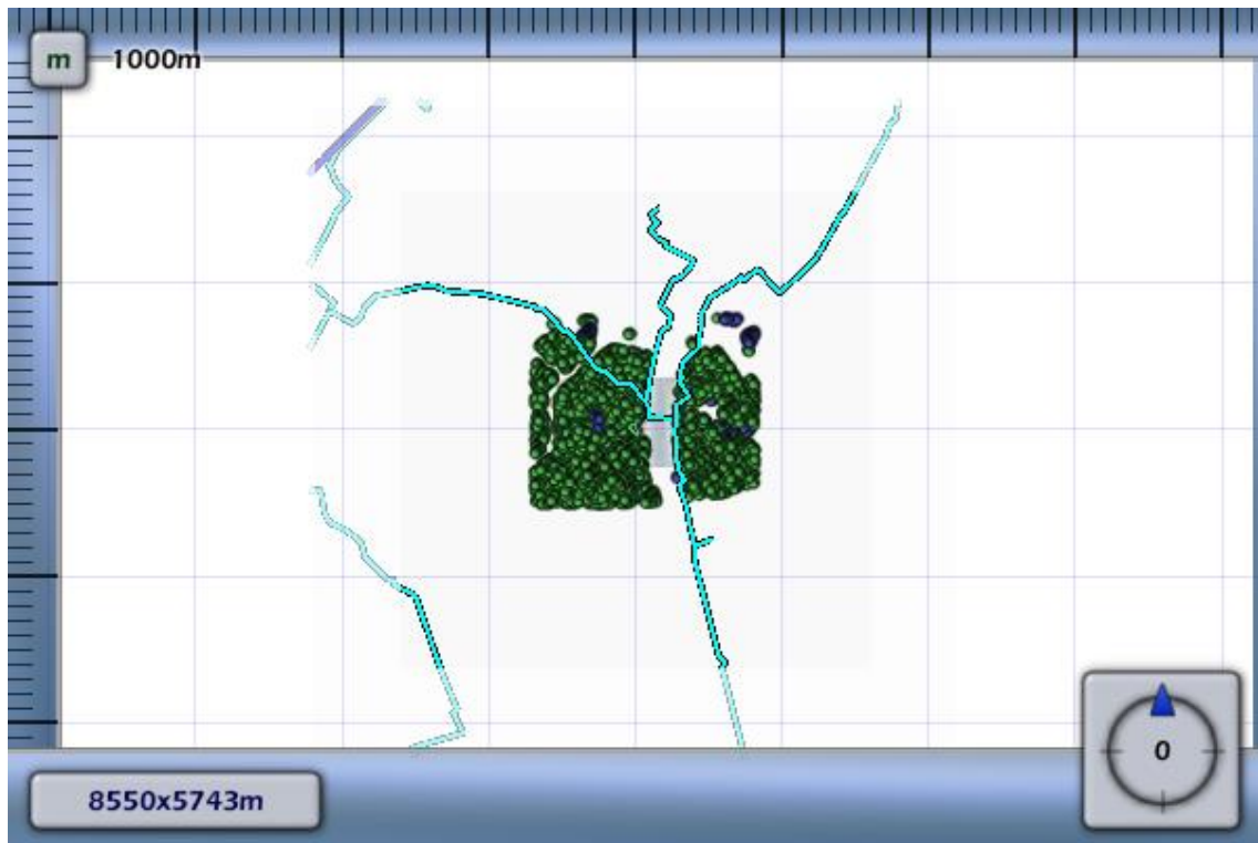
4.3 Figuur 4.3 Groepsrisico screening voor 6344_leiding-A-663-deel-1 van N.V. Nederlandse Gasunie
