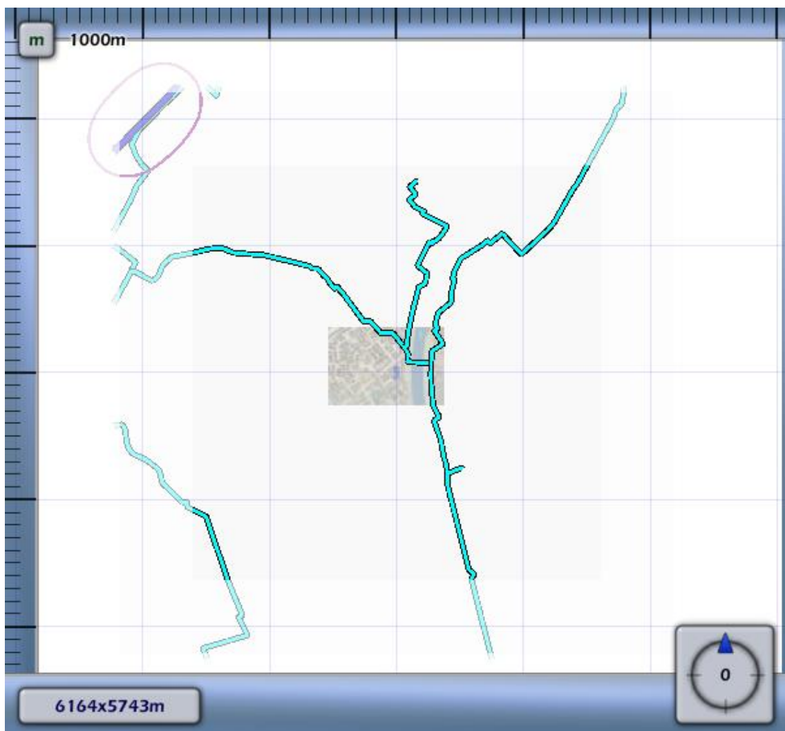
3.1 Figuur 3.1 Plaatsgebonden risico voor 6344_leiding-A-524-deel-1 van N.V. Nederlandse Gasunie
