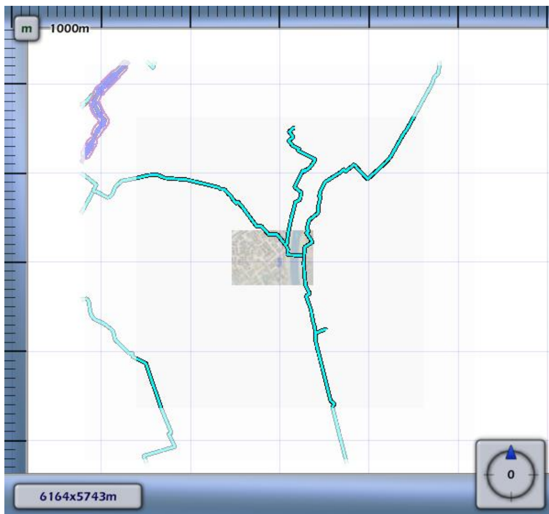
3.5 Figuur 3.5 Plaatsgebonden risico voor 6344_leiding-N-576-01-deel-2 van N.V. Nederlandse Gasunie
