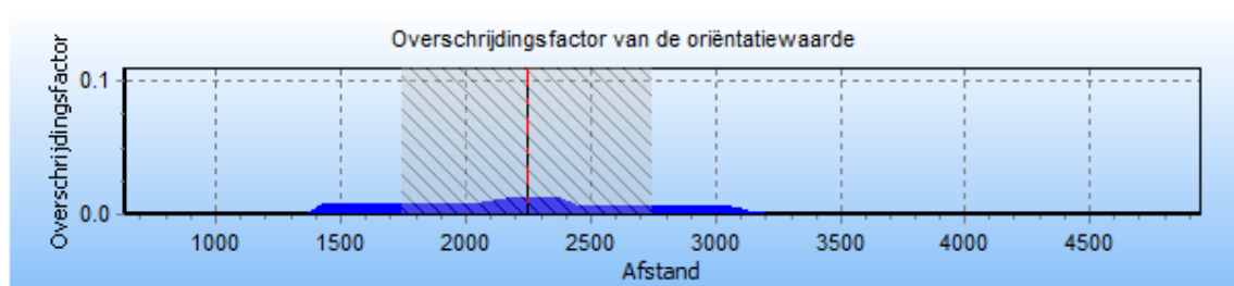
4.8 Figuur 4.8 Groepsrisico screening voor 6344_leiding-N-576-67-deel-1 van N.V. Nederlandse Gasunie
