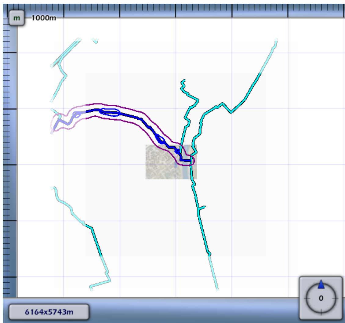
3.7 Figuur 3.7 Plaatsgebonden risico voor 6344_leiding-N-576-02-deel-1 van N.V. Nederlandse Gasunie
