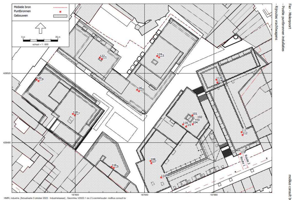
Figuur 5: Model met positie bronnen installaties en laden en lossen
