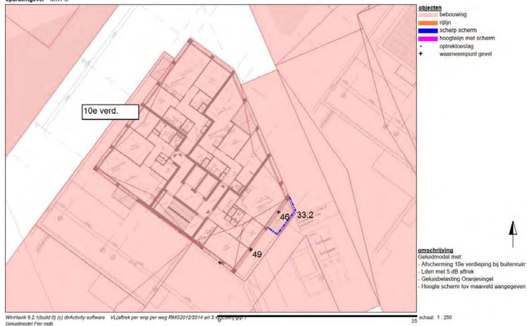
Figuur 12: Geluidsbelasting Oranjesingel 10e verdieping. Lden na aftrek, inclusief balkonafscherming
