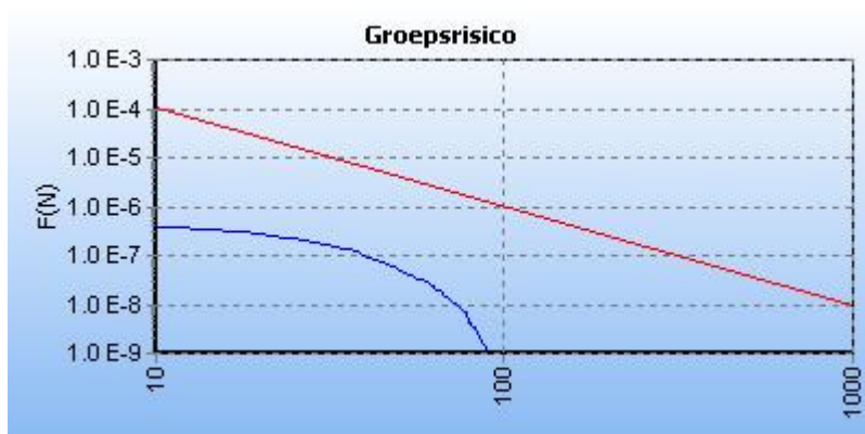
5.5 Figuur 5.5 FN curve voor N-576-02 van N.V. Nederlandse Gasunie voor de kilometer tussen stationing 2950.00 en stationing 3950.00
