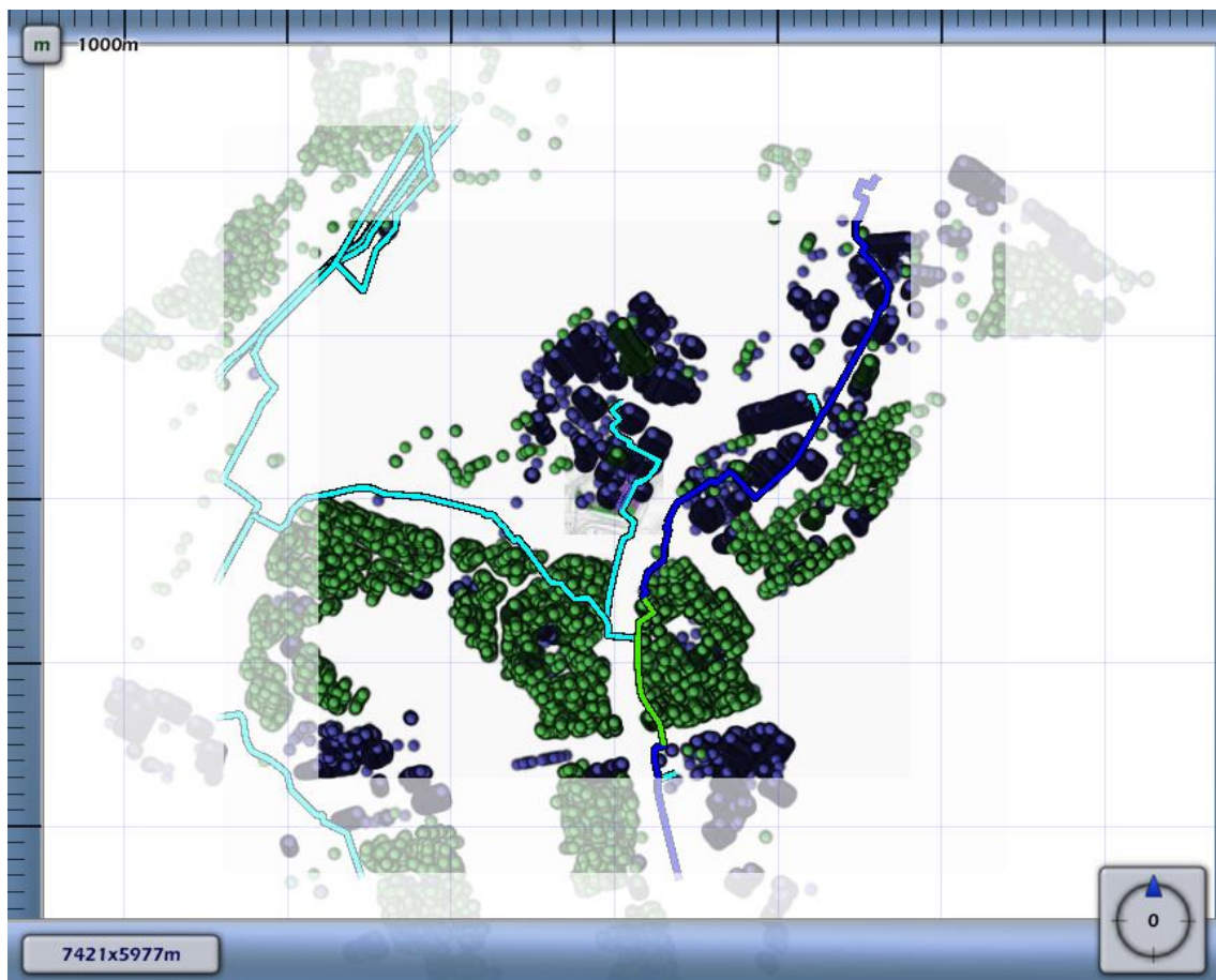
4.9 Figuur 4.9 Groepsrisico screening voor N-576-68 van N.V. Nederlandse Gasunie
