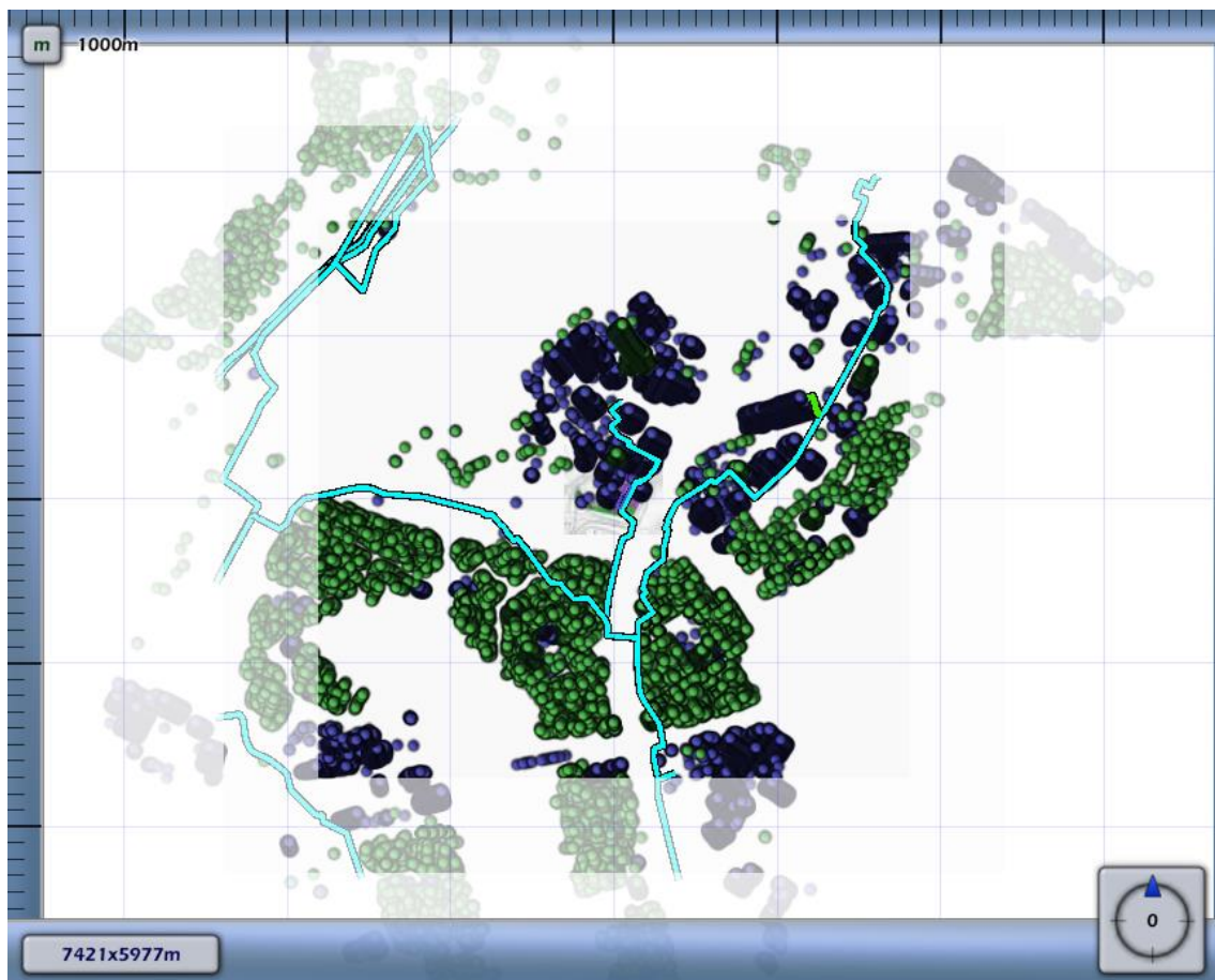
4.8 Figuur 4.8 Groepsrisico screening voor N-576-67 van N.V. Nederlandse Gasunie
