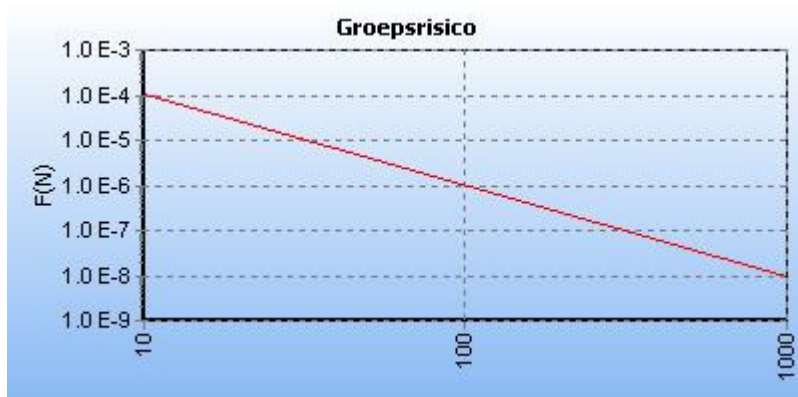
5.11 Figuur 5.11 FN curve voor N-576-70 van N.V. Nederlandse Gasunie voor de kilometer tussen stationing 0.00 en stationing 0.00
