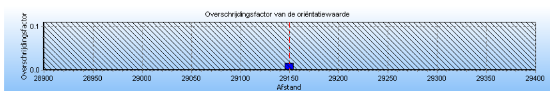
4.2 Figuur 4.2 Groepsrisico screening voor A-533 van N.V. Nederlandse Gasunie
