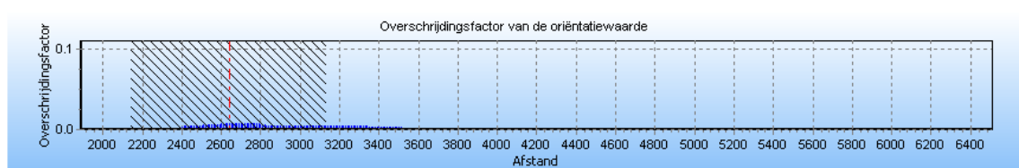
4.8 Figuur 4.8 Groepsrisico screening voor N-576-67 van N.V. Nederlandse Gasunie
