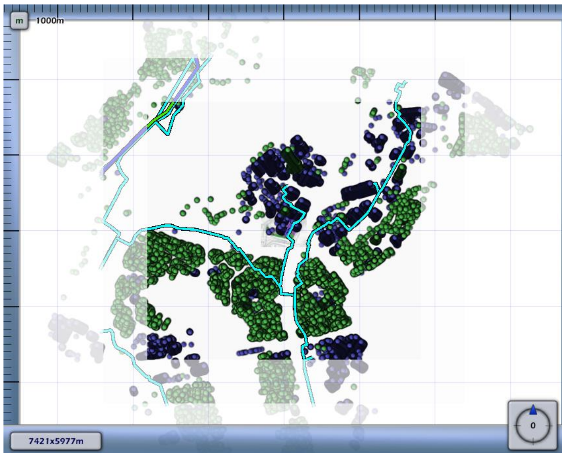
4.2 Figuur 4.2 Groepsrisico screening voor A-533 van N.V. Nederlandse Gasunie
