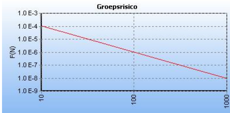
5.10 Figuur 5.10 FN curve voor N-576-69 van N.V. Nederlandse Gasunie voor de kilometer tussen stationing 10.00 en stationing 110.00
