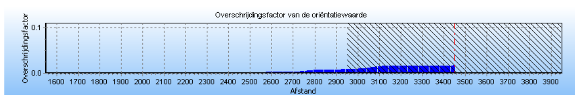
4.5 Figuur 4.5 Groepsrisico screening voor N-576-02 van N.V. Nederlandse Gasunie
