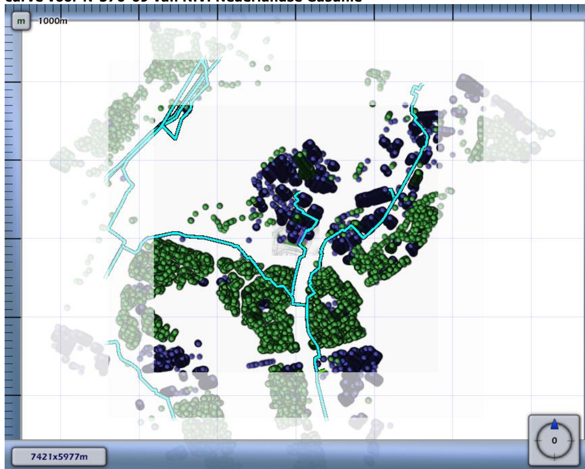
Figuur 4.10 Kilometer leiding behorende bij de maximale overschrijding van de FN-curve voor N-576-69 van N.V. Nederlandse Gasunie
