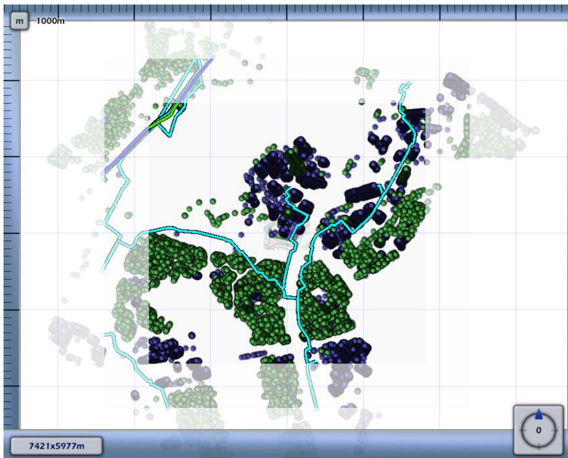
4.4 Figuur 4.4 Groepsrisico screening voor N-576-01 van N.V. Nederlandse Gasunie
