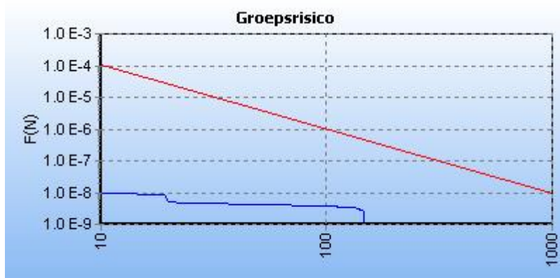
5.4 Figuur 5.4 FN curve voor N-576-01 van N.V. Nederlandse Gasunie voor de kilometer tussen stationing 2870.00 en stationing 3760.00
