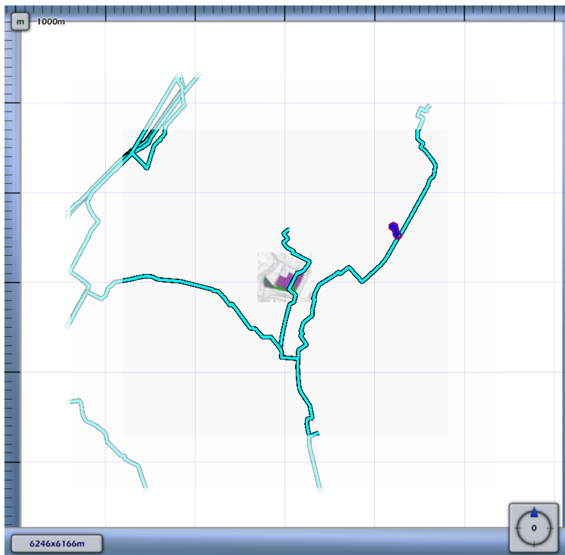
3.7 Figuur 3.7 Plaatsgebonden risico voor N-576-66 van N.V. Nederlandse Gasunie
