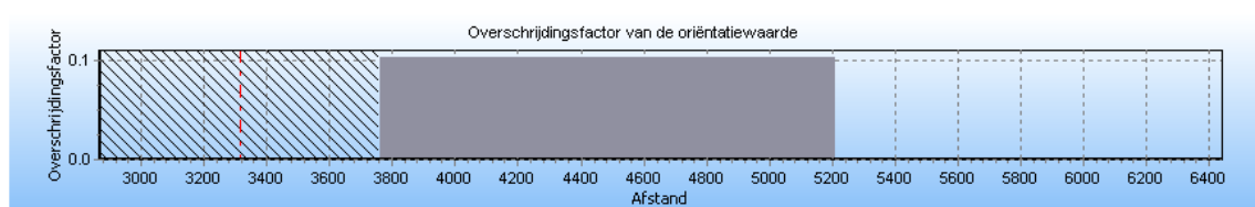
4.4 Figuur 4.4 Groepsrisico screening voor N-576-01 van N.V. Nederlandse Gasunie
