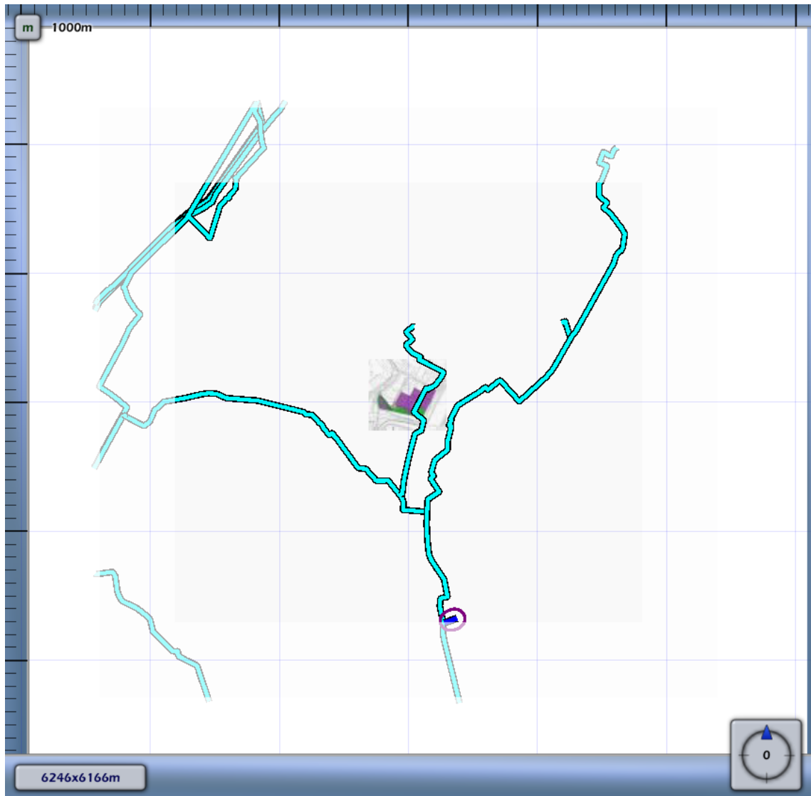
3.10 Figuur 3.10 Plaatsgebonden risico voor N-576-69 van N.V. Nederlandse Gasunie
