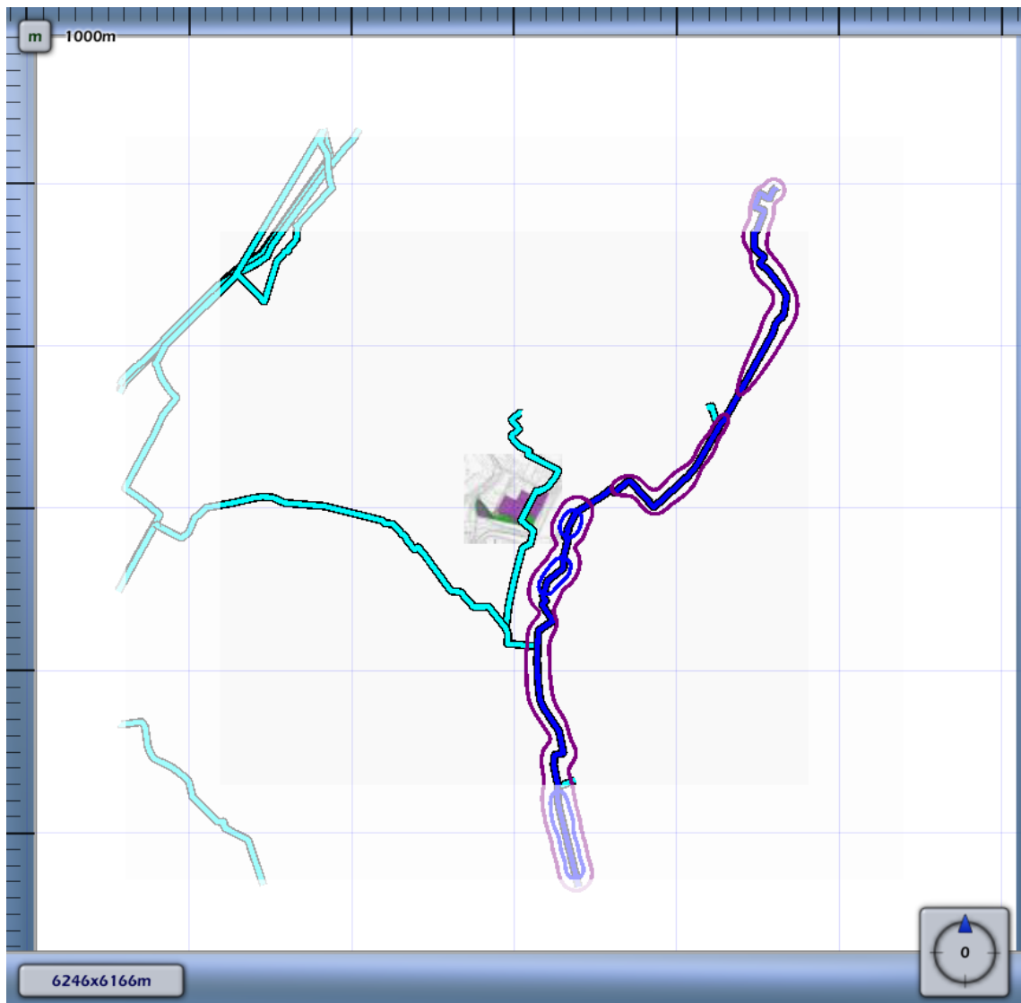
3.8 Figuur 3.8 Plaatsgebonden risico voor N-576-67 van N.V. Nederlandse Gasunie
