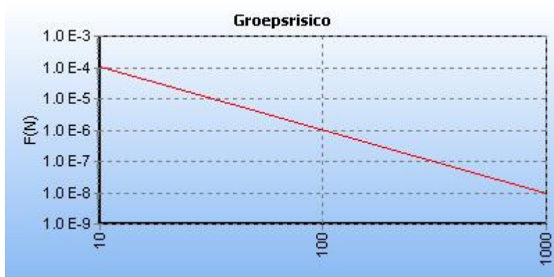
5.8 Figuur 5.8 FN curve voor N-576-67 van N.V. Nederlandse Gasunie voor de kilometer tussen stationing 2140.00 en stationing 3140.00
