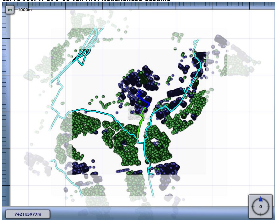
Figuur 4.9 Kilometer leiding behorende bij de maximale overschrijding van de FN-curve voor N-576-68 van N.V. Nederlandse Gasunie
