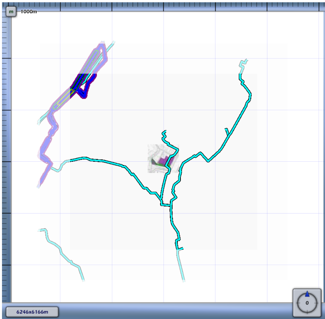
3.4 Figuur 3.4 Plaatsgebonden risico voor N-576-01 van N.V. Nederlandse Gasunie
