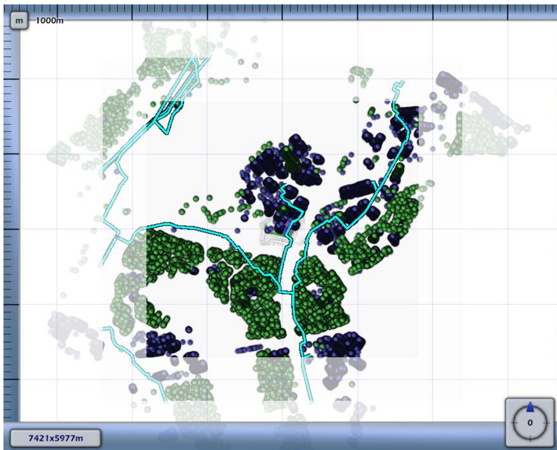
4.7 Figuur 4.7 Groepsrisico screening voor N-576-66 van N.V. Nederlandse Gasunie
