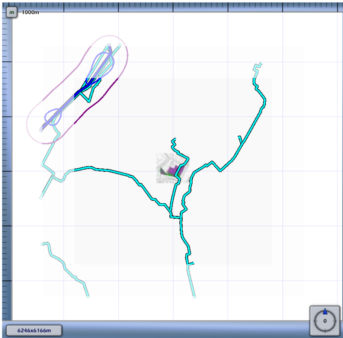
3.1 Figuur 3.1 Plaatsgebonden risico voor A-524 van N.V. Nederlandse Gasunie
