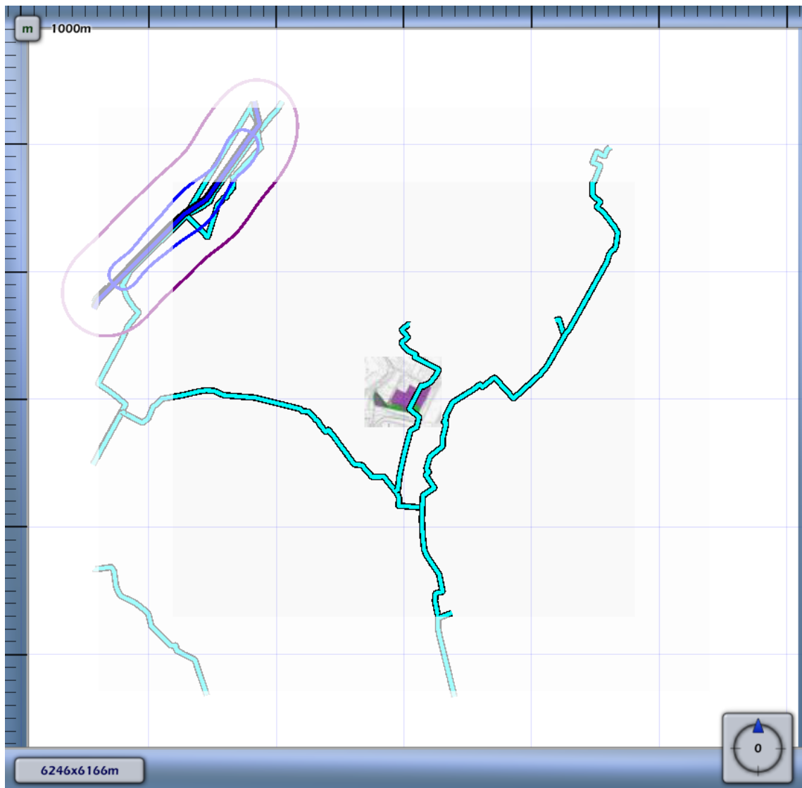
3.2 Figuur 3.2 Plaatsgebonden risico voor A-533 van N.V. Nederlandse Gasunie
