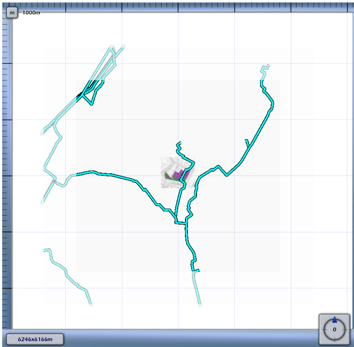
3.6 Figuur 3.6 Plaatsgebonden risico voor N-576-04 van N.V. Nederlandse Gasunie
