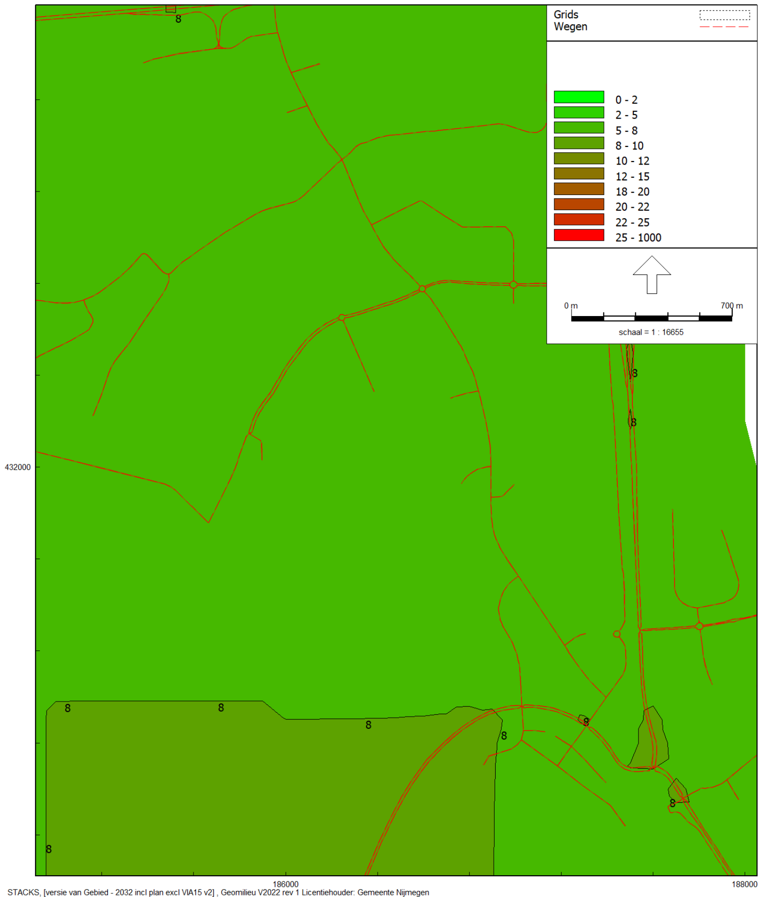
Figuur overzicht 2032 incl plan geen VIA15 concentraties ug/m3 PM2,5
