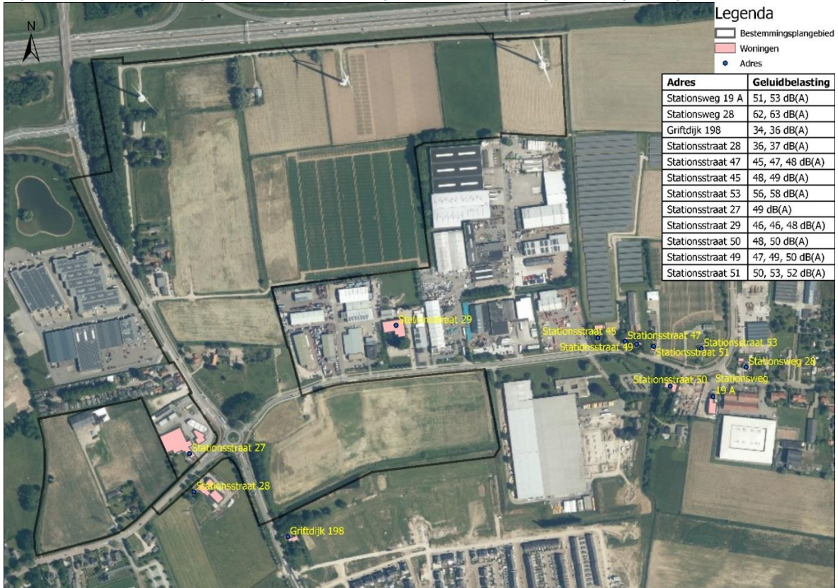
Figuur 5.6a: Geluidbelasting van het bestaande bedrijventerrein in de huidige situatie (HS_BB).
