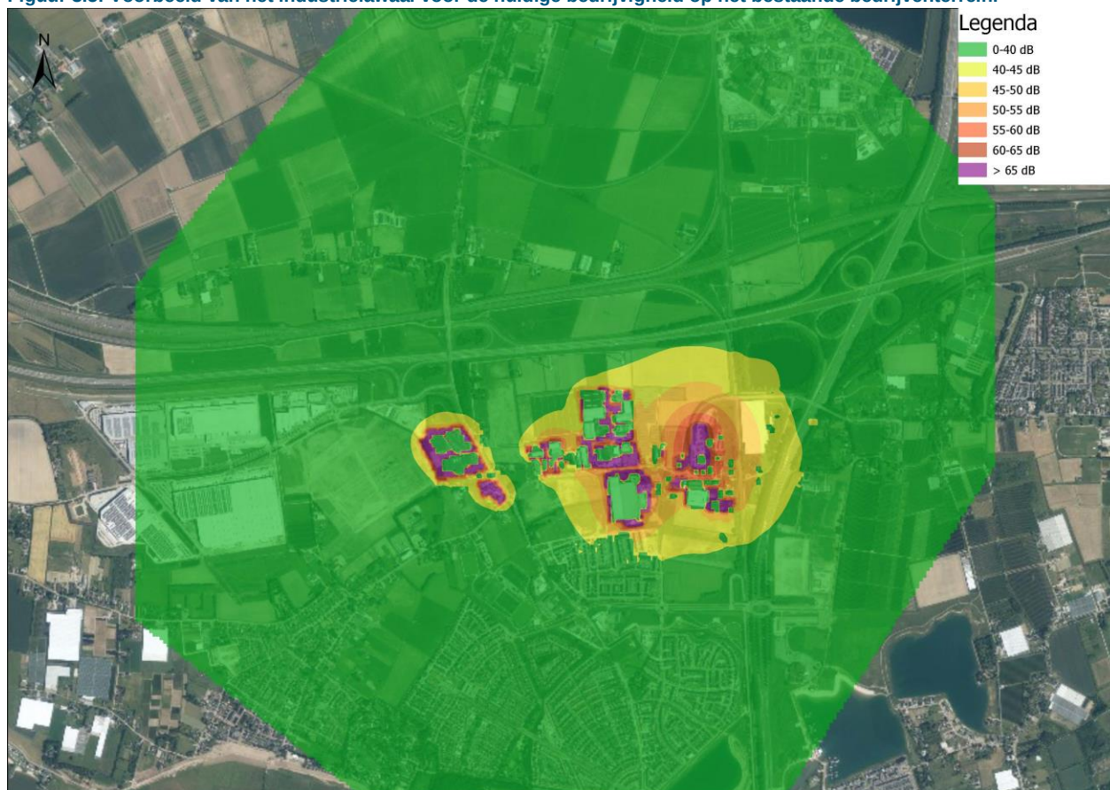
Figuur 3.5: Voorbeeld van het industrielawaai voor de huidige bedrijvigheid op het bestaande bedrijventerrein.
