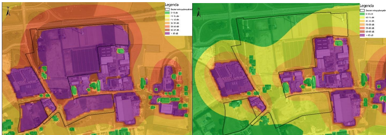
Figuur 5.3a: Geluidbelasting L_{etmaal} voor het industrielaawaai voor de maximale planologische situatie in de vorm van contouren op een hoogte van 5 meter. Links het uitgebreide bedrijventerrein en rechts het bestaande terrein.
