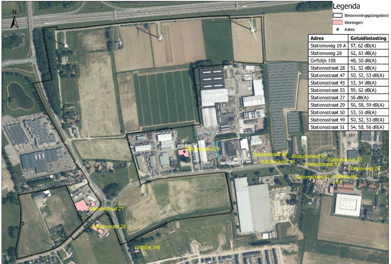
Figuur 5.6c: Geluidbelasting van het bestaande en toekomstige bedrijventerrein voor de maximale planologische situatie (TS_BB_en_NB_MS).
