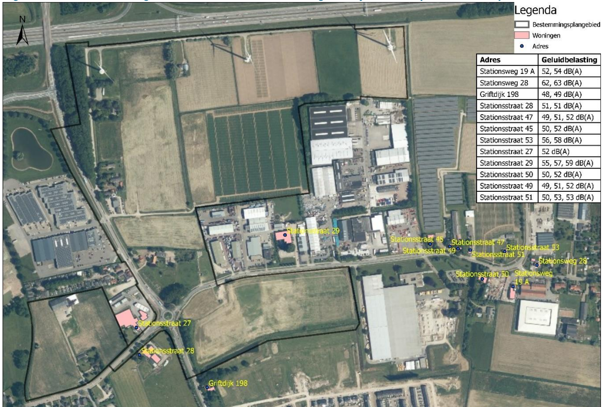
Figuur 5.6b: Geluidbelasting van het bestaande en toekomstige bedrijventerrein (TS_BB en NB).
