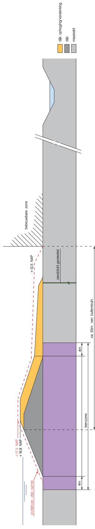
profiel 1e zanddicht geotextiel + steunberm
