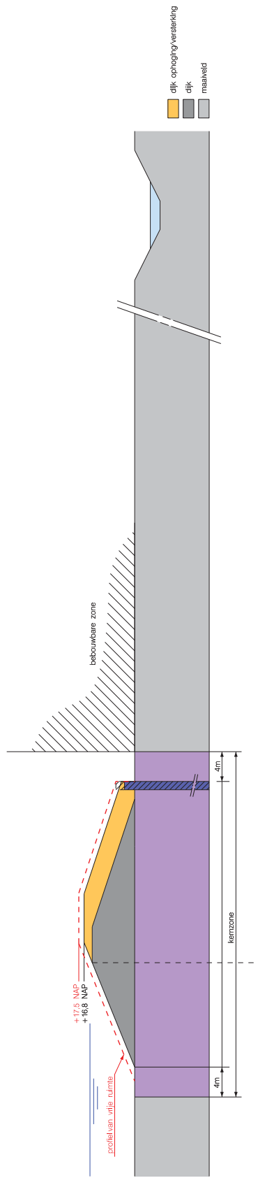
profiel 1d Constructief kwelscherm
