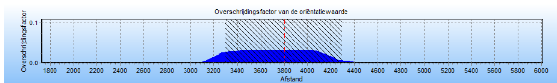
4.4 Figuur 4.4 Groepsrisico screening voor 1107_leiding-A-524-deel-1 van N.V. Nederlandse Gasunie
