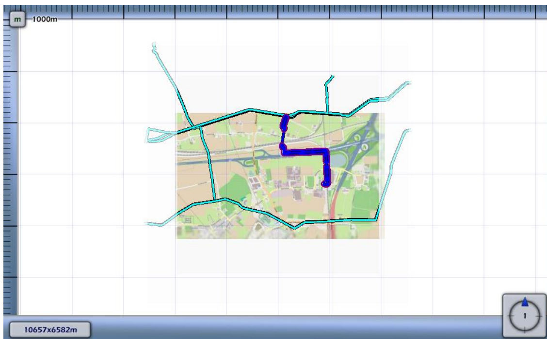
3.11 Figuur 3.11 Plaatsgebonden risico voor 1107_leiding-N-578-19-deel-1 van N.V. Nederlandse Gasunie
