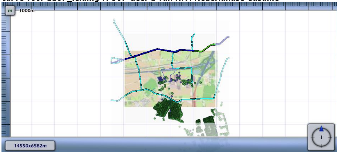
Figuur 4.2 Kilometer leiding behorende bij de maximale overschrijding van de FN-curve voor 1107_leiding-A-507-deel-1 van N.V. Nederlandse Gasunie
