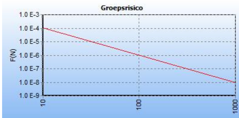
5.11 Figuur 5.11 FN curve voor 1107_leiding-N-578-19-deel-1 van N.V. Nederlandse Gasunie voor de kilometer tussen stationing 0.00 en stationing 1000.00
