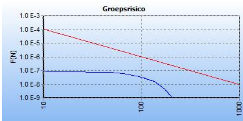
5.5 Figuur 5.5 FN curve voor 1107_leiding-A-533-deel-1 van N.V. Nederlandse Gasunie voor de kilometer tussen stationing 3320.00 en stationing 4320.00
