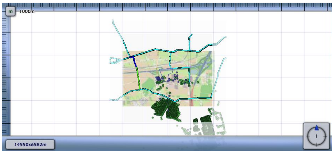
4.4 Figuur 4.4 Groepsrisico screening voor 1107_leiding-A-524-deel-1 van N.V. Nederlandse Gasunie
