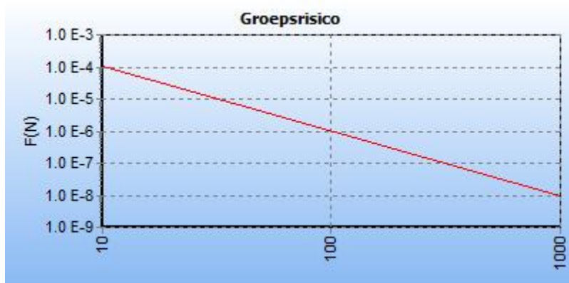
5.12 Figuur 5.12 FN curve voor 1107_leiding-N-578-20-deel-1 van N.V. Nederlandse Gasunie voor de kilometer tussen stationing 0.00 en stationing 1000.00
