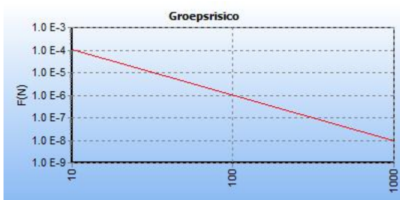
5.8 Figuur 5.8 FN curve voor 1107_leiding-N-568-37-deel-1 van N.V. Nederlandse Gasunie voor de kilometer tussen stationing 0.00 en stationing 680.00
