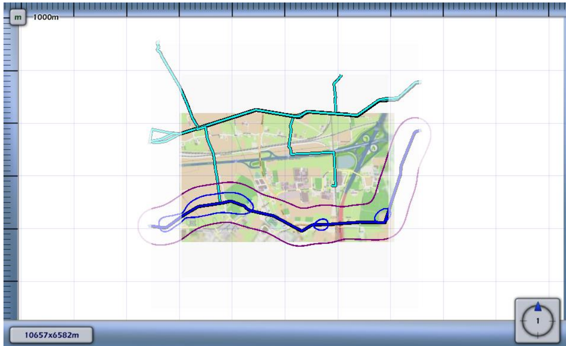
3.5 Figuur 3.5 Plaatsgebonden risico voor 1107_leiding-A-533-deel-1 van N.V. Nederlandse Gasunie
