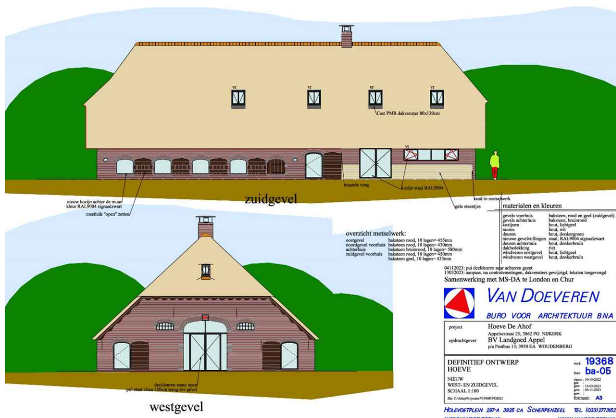
Afbeelding 10: nieuwe situatie zuid- en westgevel Restauratieplan De Ahof Bron: Van Doeveren buro voor architectuur
