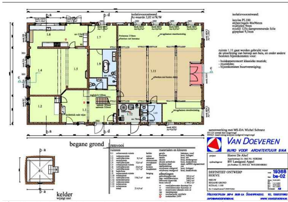
Afbeelding 11: plattegrond nieuwe situatie begane grond Restauratieplan Ahof Bron: Van Doeveren buro voor architectuur
