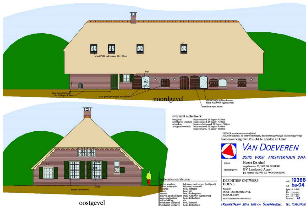
Afbeelding 9: nieuwe noord- en oostgevel Restauratieplan De Ahof Bron: Van Doeveren bureau voor architectuur
