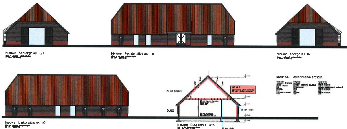
Afbeelding 5: Gevelaanzichten van de nieuwe situatie
