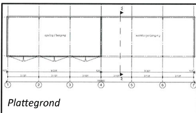
Figuur 9: plattegrondtekening bijgebouw, werktuigenberging
