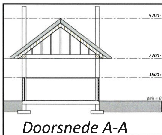
Figuur 4: doorsnedetekening bijgebouw, hooiberg
