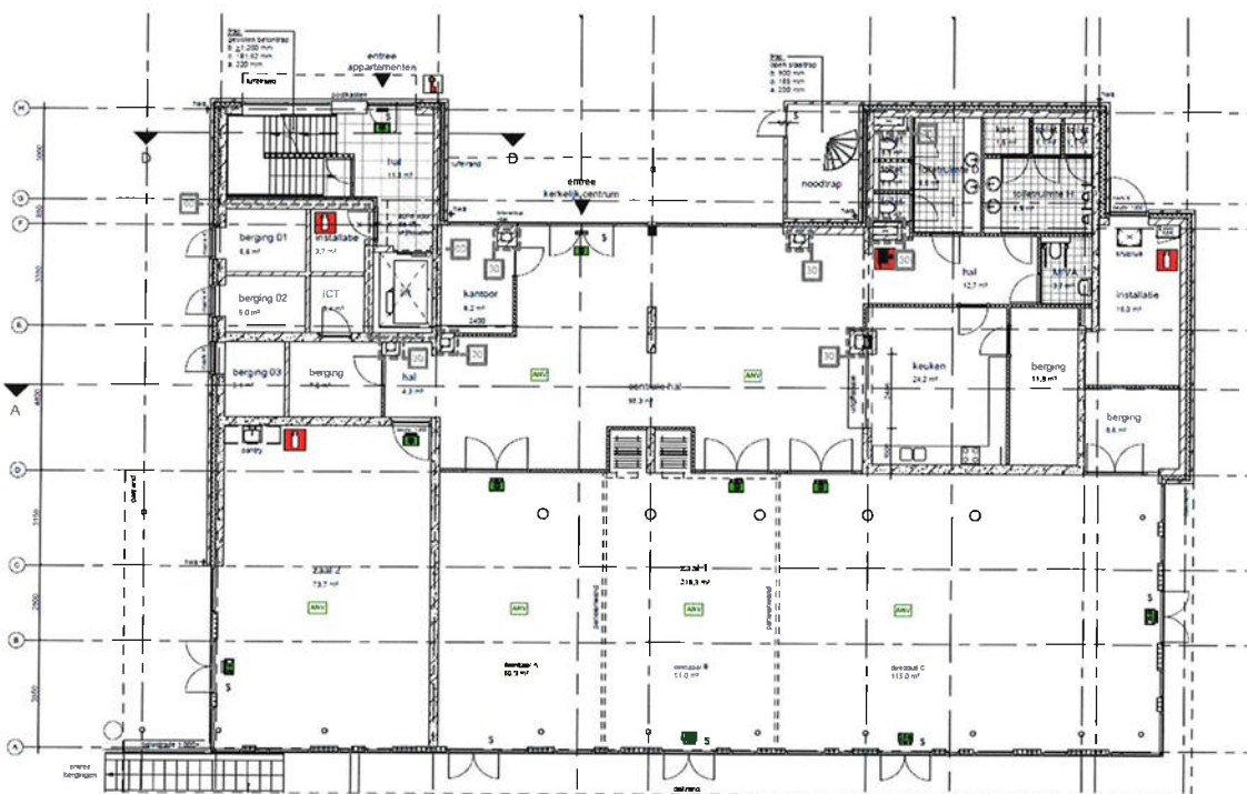
Plattegrond begane grond (kerkelijk centrum)
