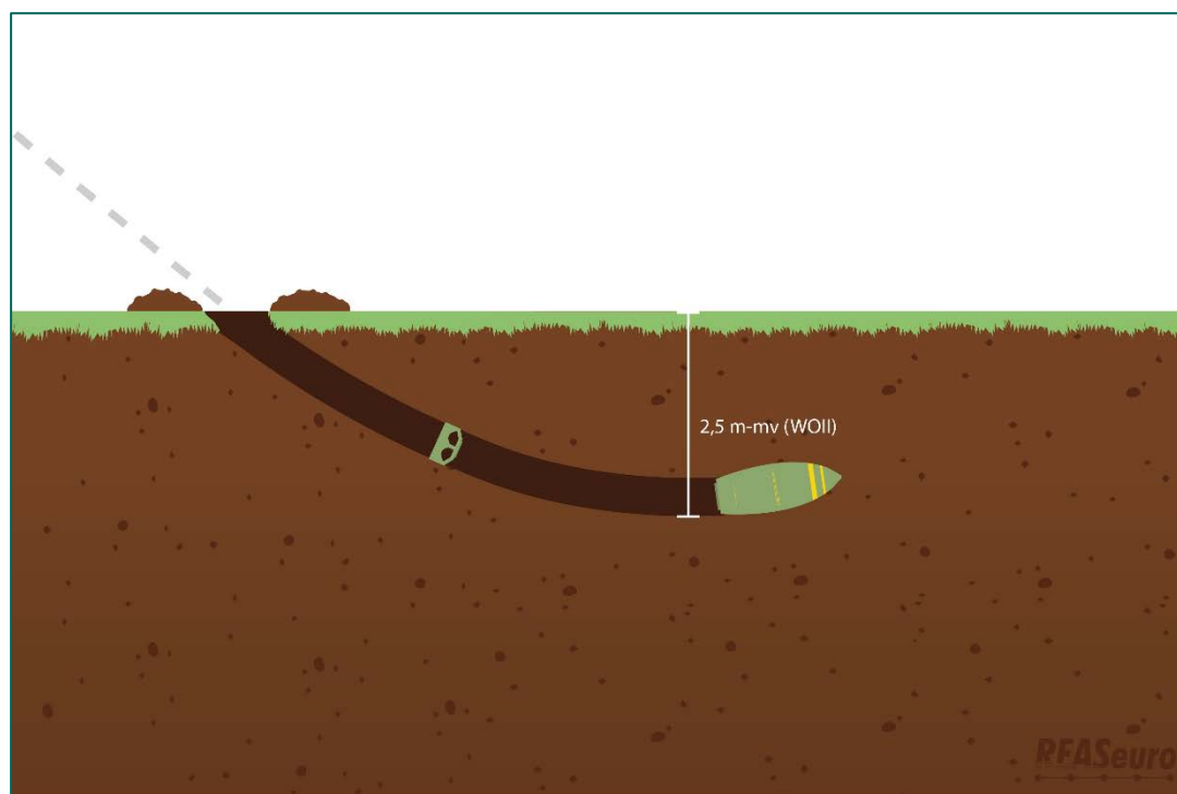
Figuur 8. Schematische weergave van indringing van een projectiel met de maximale penetratiediepte.
