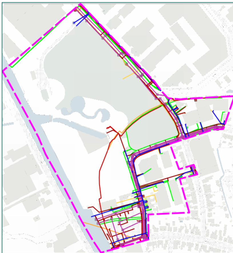
Figuur 50. Overzicht van de kabels en leidingen binnen de projectlocatie (bron: Klic).
