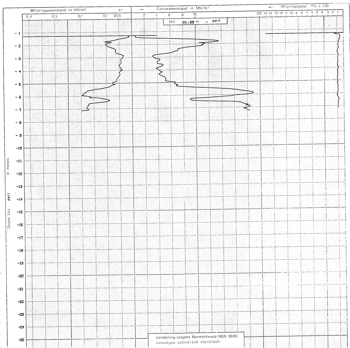
Figuur 46. Sondering S32E00084 d.d. 21-06-1979 (bron gegevens: Dinoloket).
