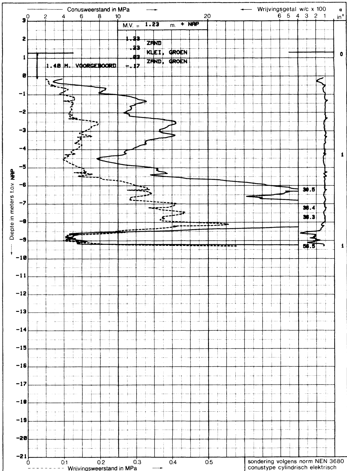
Figuur 47. Sondering S32E00020 d.d. 01-01-1992 (bron gegevens: Dinoloket).
