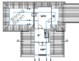
Best. Verdieping 188 m² vloeroppervlakte 12 m²
