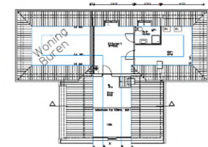
Nieuwe Verdieping 188 m² vloeroppervlakte 12 m²
