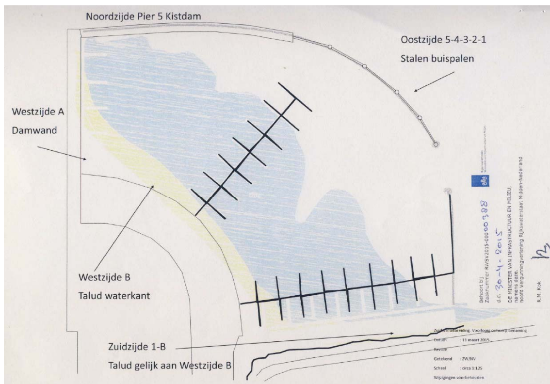
Figuur 3.1 Tekening van het initiatief
