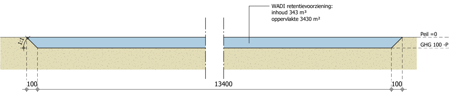
DOORSNEDE WADI RETENTIEVOORZIENING (1:20)
