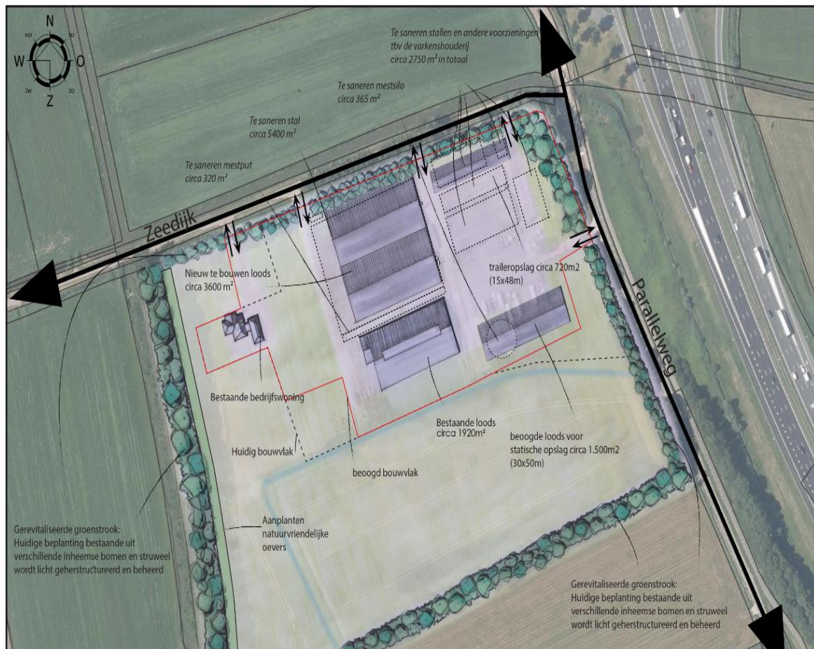
Stedenbouwkundig en landschappelijk inpassingsplan. Bron: Van Dun Advies.
