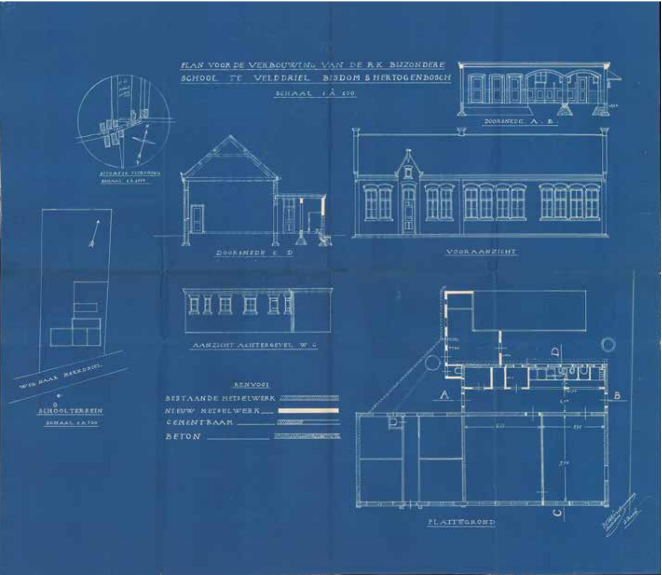
1933 tekening tbv verbouwing
