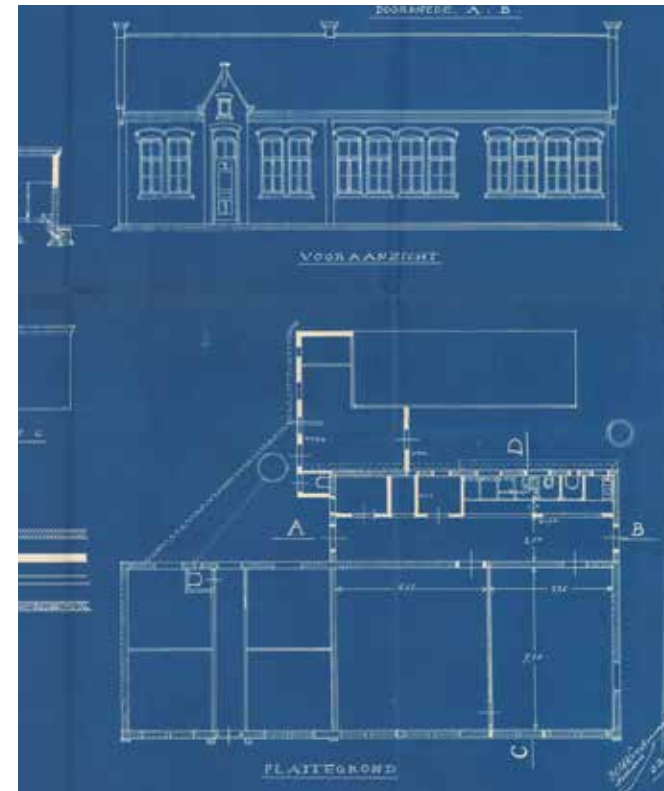
detail bouwvergunning 1933, de nieuw gebouwde delen zijn in wit aangegeven (RAR 3113-03336_0009)
