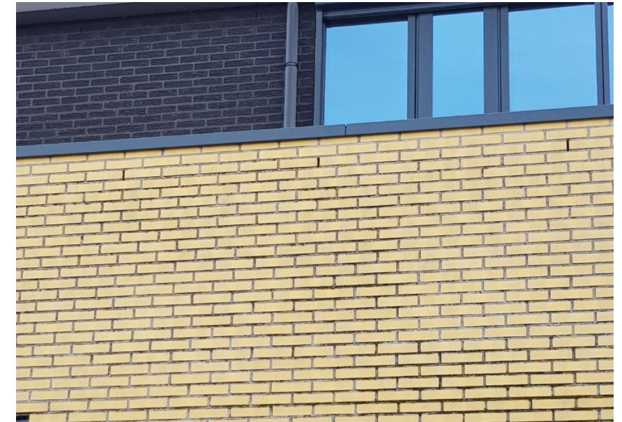
Figuur 10: Open stootvoegen in de gevel van het bedrijfsgebouw
