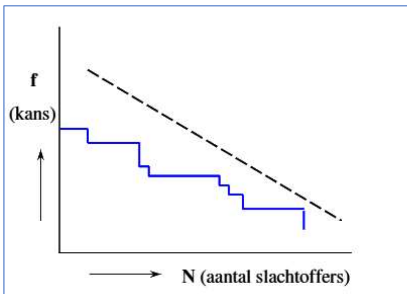
Afbeelding 2.1: voorbeeld FN curve met de oriëntatiewaarde als stippellijn weergegeven
