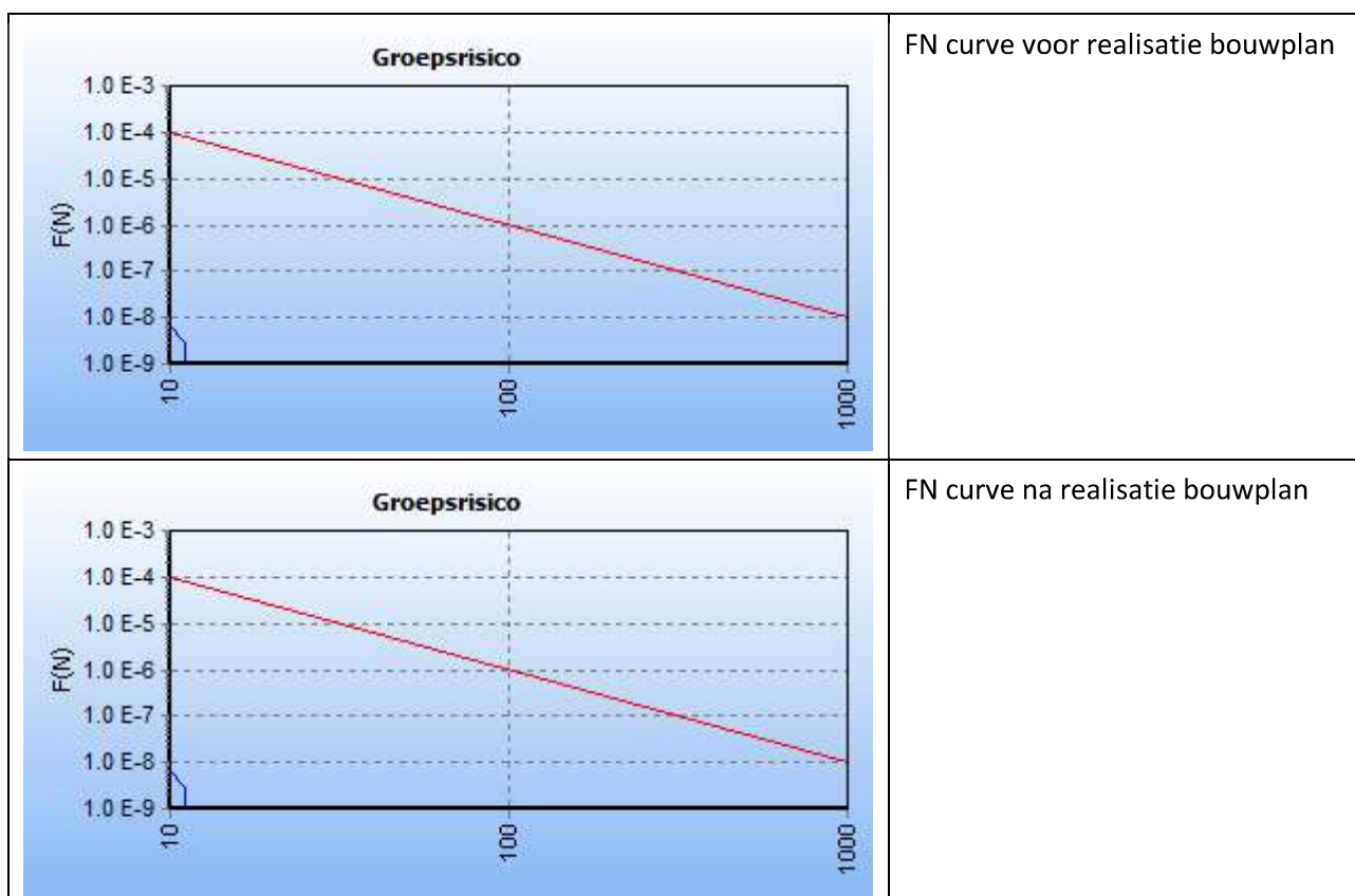
Afbeelding 4.2: FN curves voor en na realisatie bouwplan
