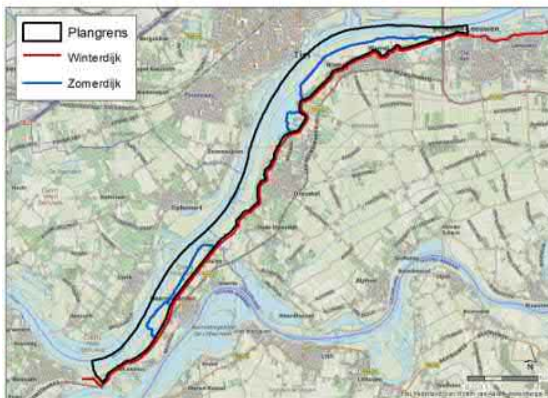
Figuur 11.7 Ligging van de winter- en zomerdijk
