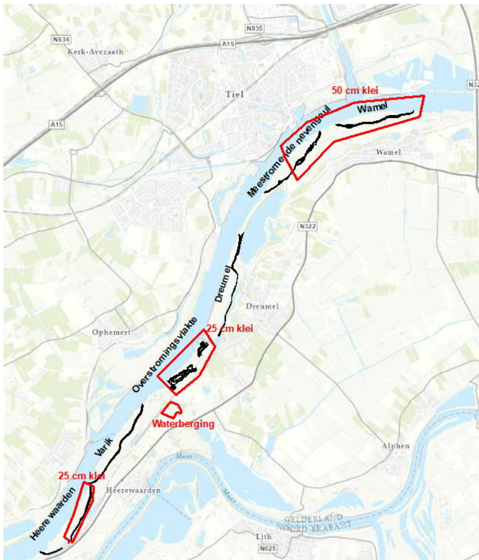
Abbeelding 11.13. locaties met kleilagen ter mitigatie van geohydrologische effecten
