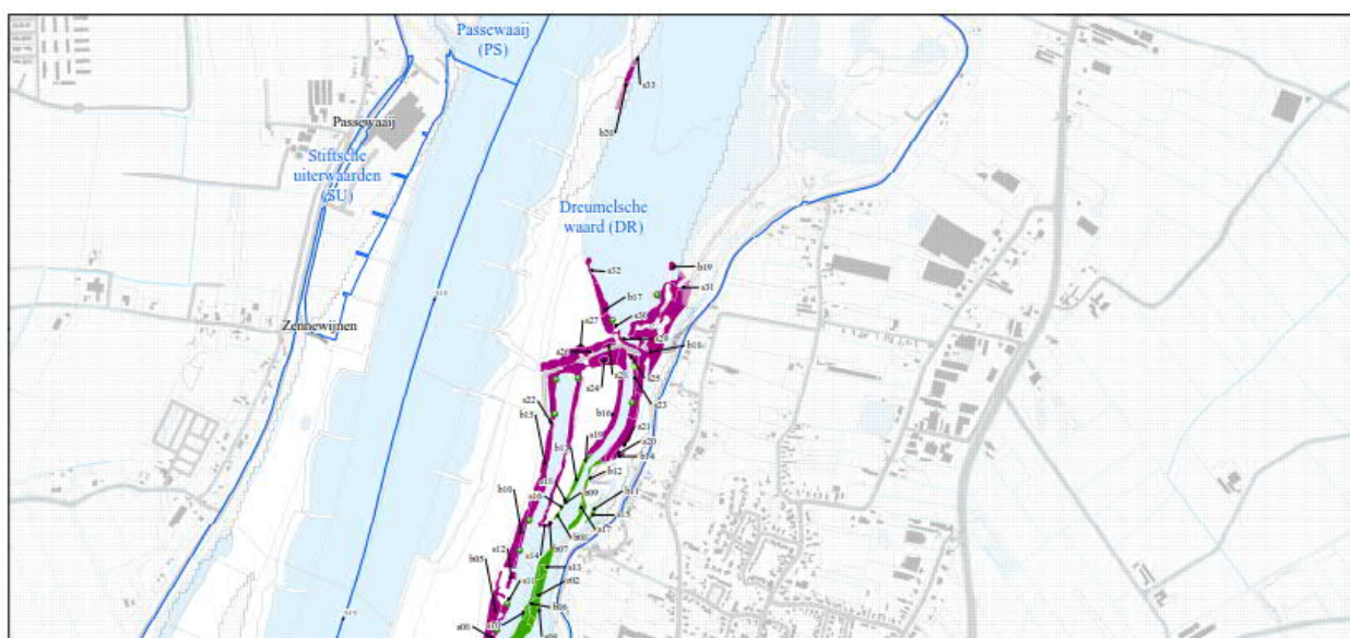
Afbeelding 3.2: Overzicht te verwijderen bosschages vanuit programma Stroomlijn.
