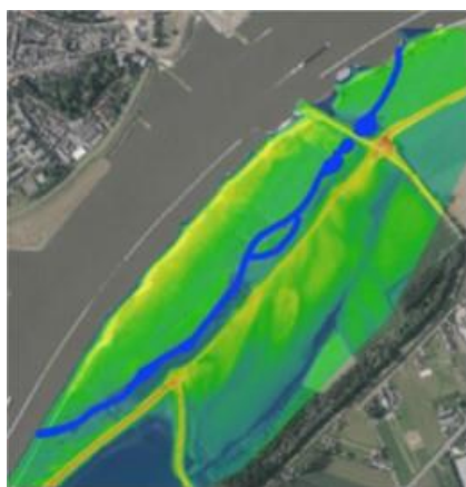
Figuur 2.3: Tracé van de permanent stromende nevengeul weergegeven op de hoogtekarta van de huidige situatie (links) en dwarsdoorsnede permanent stromende nevengeul bij de Tielse Plaat. De doorsnede is van een traject stroomafwaarts van het inlaatwerk (rechts).
