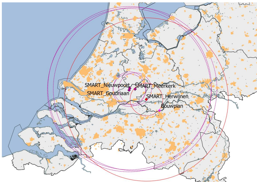
Figuur 5 Locaties van de drie alternatieve locaties Goudriaan, Meerkerk en Nieuwpoort (paarse ruit) voor de nieuwe SMART-L EWC GB gevechtsleidingsradar te Herwijnen (rode ruit). De oranje vlakken zijn de in de AHN-1 gedefinieerde stedelijke gebieden. De ligging van het te toetsen bouwplan is aangegeven met een roze ster.
