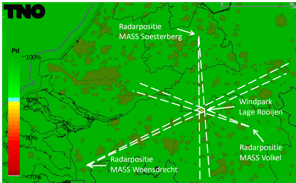
Figuur 11 Detectiekans van het primaire verkeersleidingsradarnetwerk berekend op 1000 voet in het schaduwgebied van het bouwplan nadat deze is gerealiseerd. Op dit figuur is detectiekansmiddeling toegepast. De stippellijnen geven aan waar de schaduw kan ontstaan.
