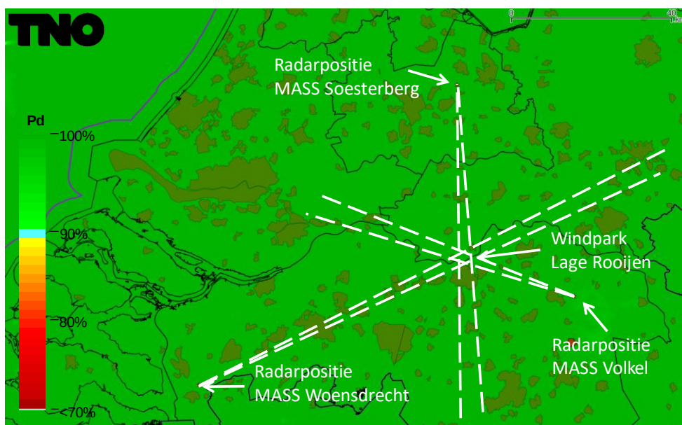
Figuur 10 Detectiekans van het primaire verkeersleidingsradarnetwerk op 1000 voet in het schaduwgebied van het bouwplan voordat deze is gerealiseerd (baseline). Op dit figuur is detectiekansmiddeling toegepast. De stippellijnen geven aan waar de schaduw kan gaan ontstaan.
