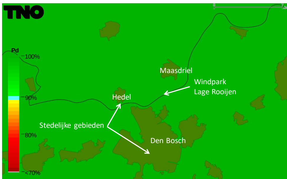
Figuur 7 Detectiekans van het primaire verkeersleidingsradarnetwerk op 1000 voet boven het bouwplan voordat dit is gerealiseerd (baseline).
