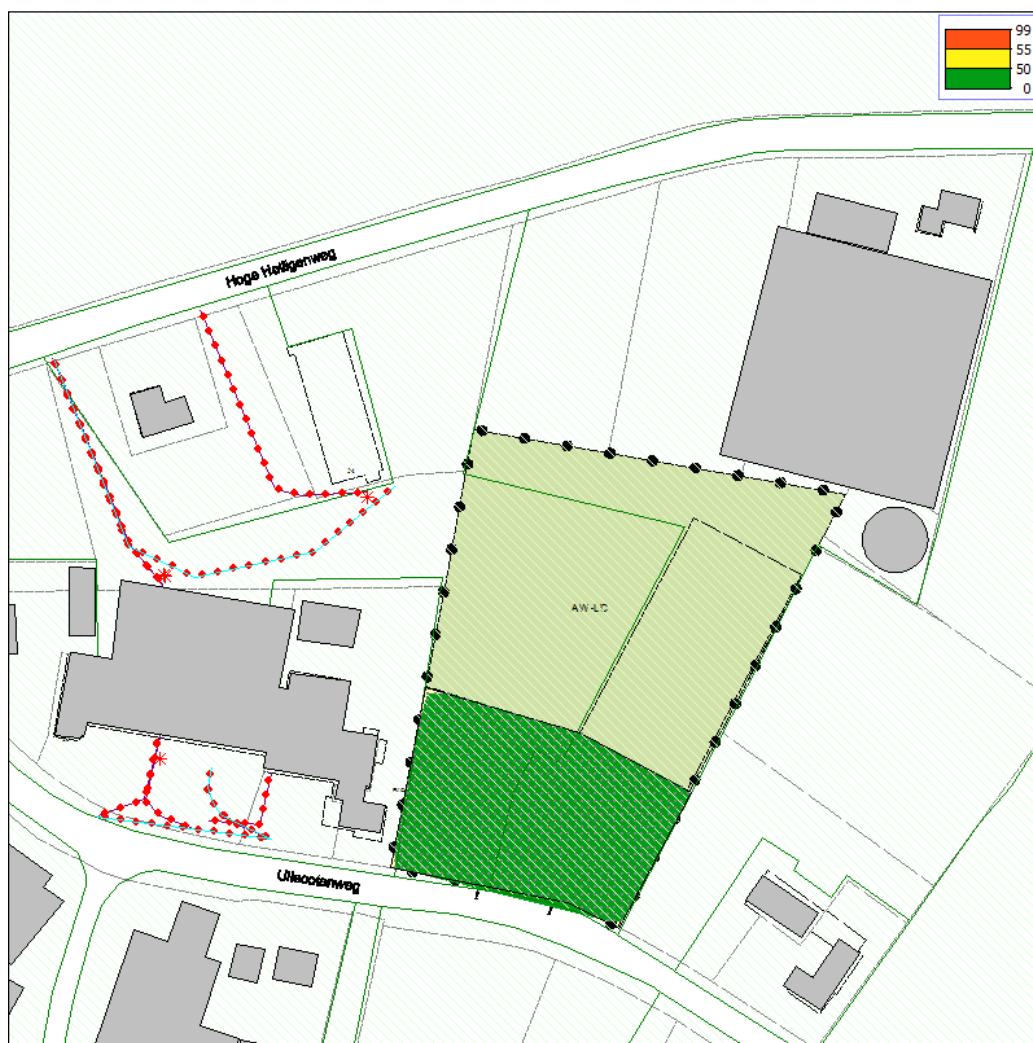
Figuur 5.2: Berekende langtijdgemiddelde beoordelingsniveaus ( L_{Ar,LT} ) in de avondperiode (rekenhoogte 5 meter) ter plaatse van plangebied 2
