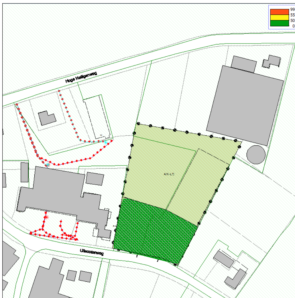
Figuur 5.3: Berekende langtijdgemiddelde beoordelingsniveaus ( L_{Ar,LT} ) in de nachtperiode (rekenhoogte 5 meter) ter plaatse van plangebied 2
