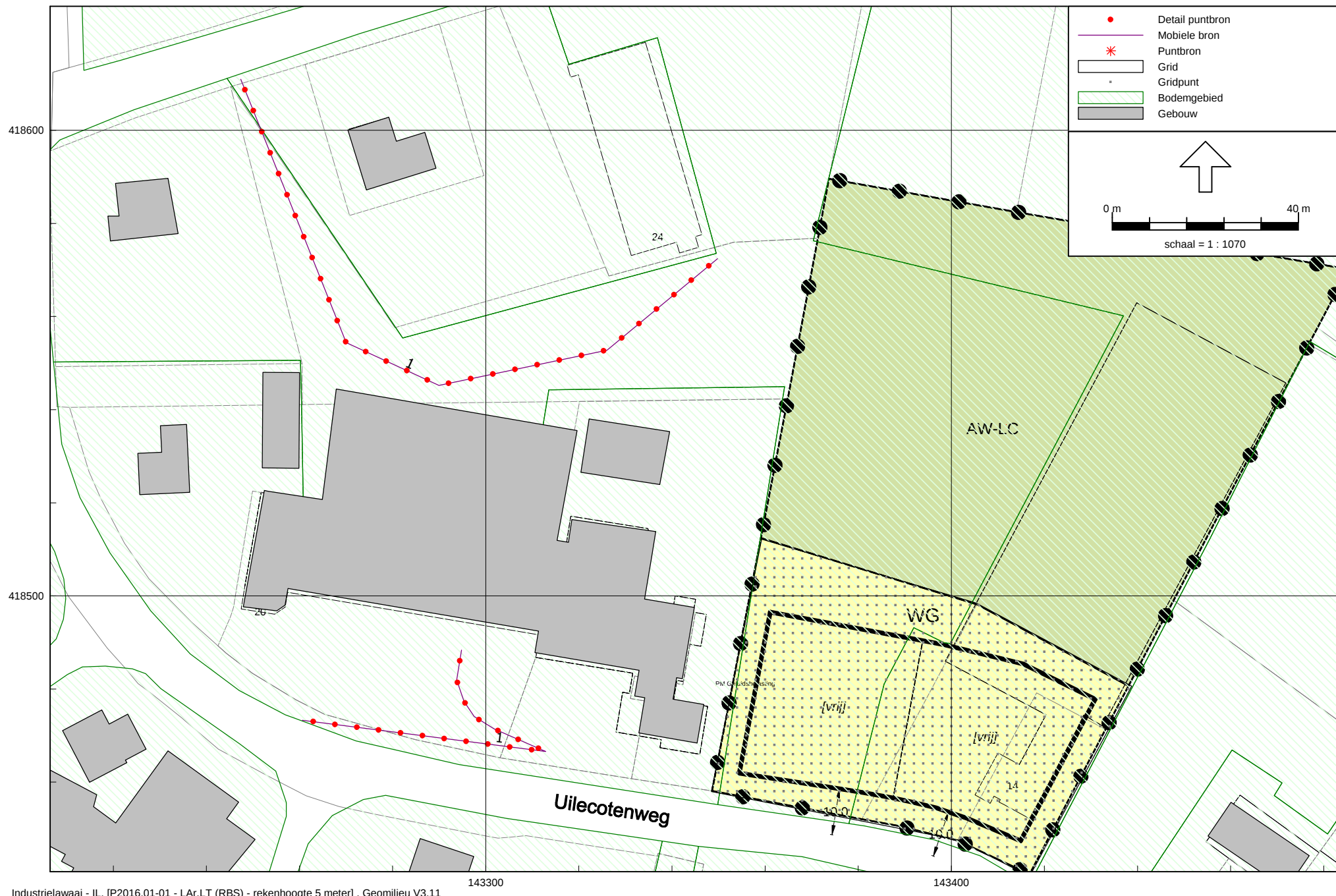
Figuur 3: Grafische weergave rekenmodel LAr,LT avondperiode - mobiele en puntbronnen
