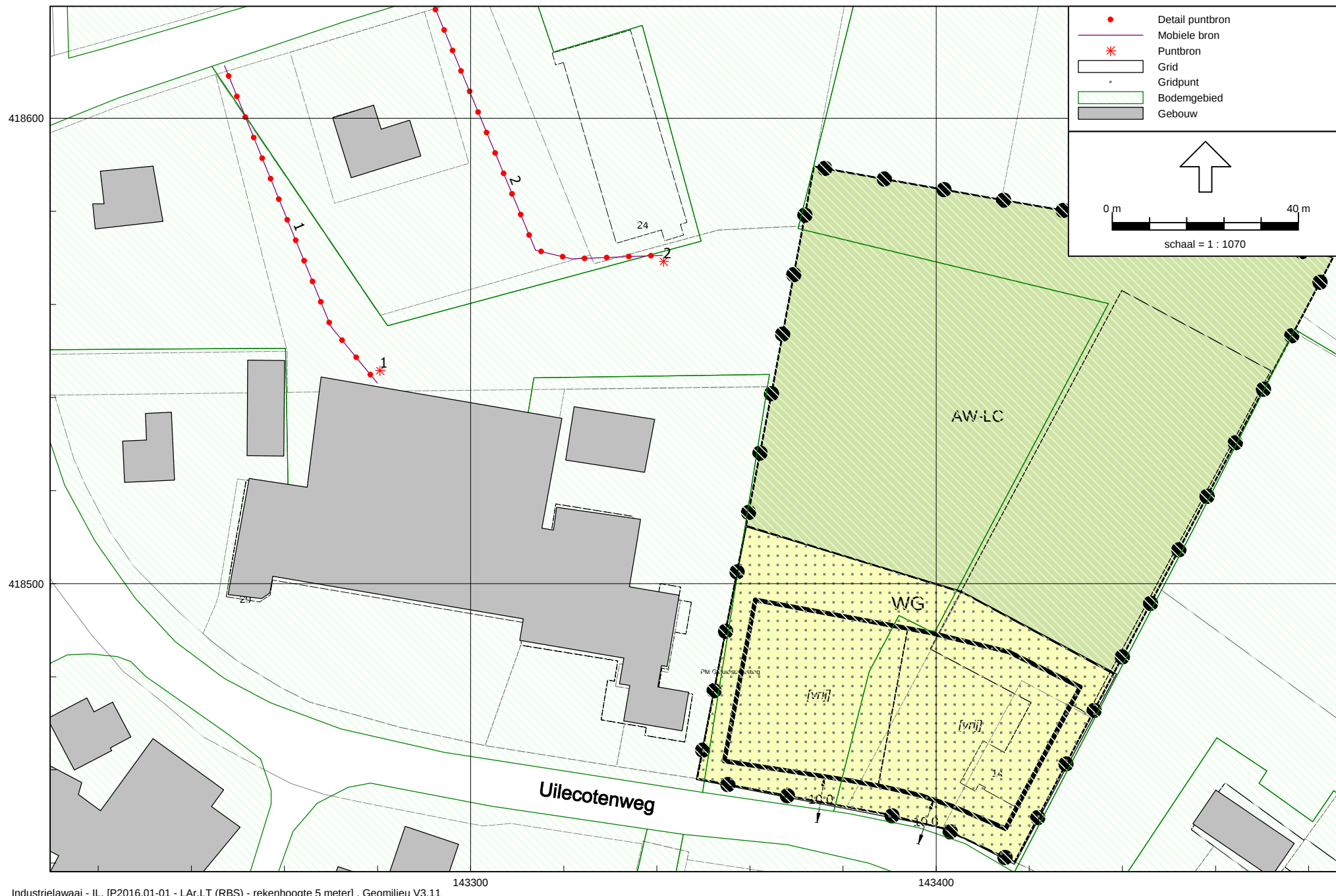
Figuur 4: Grafische weergave rekenmodel LAr,LT nachtperiode - mobiele en puntbronnen
