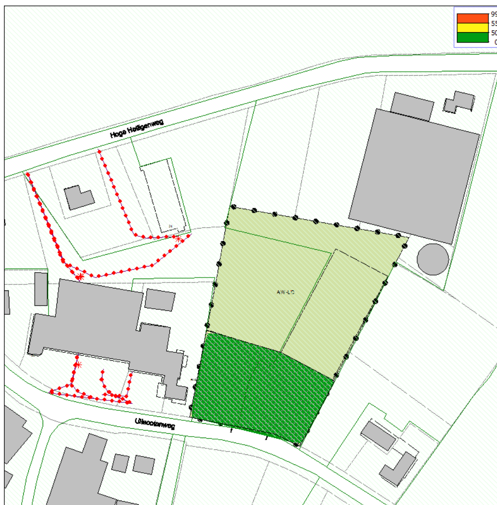
Figuur 5.1: Berekende langtijdgemiddelde beoordelingsniveaus ( L_{Ar,LT} ) in de dagperiode (rekenhoogte 1,5 meter) ter plaatse van plangebied 3
