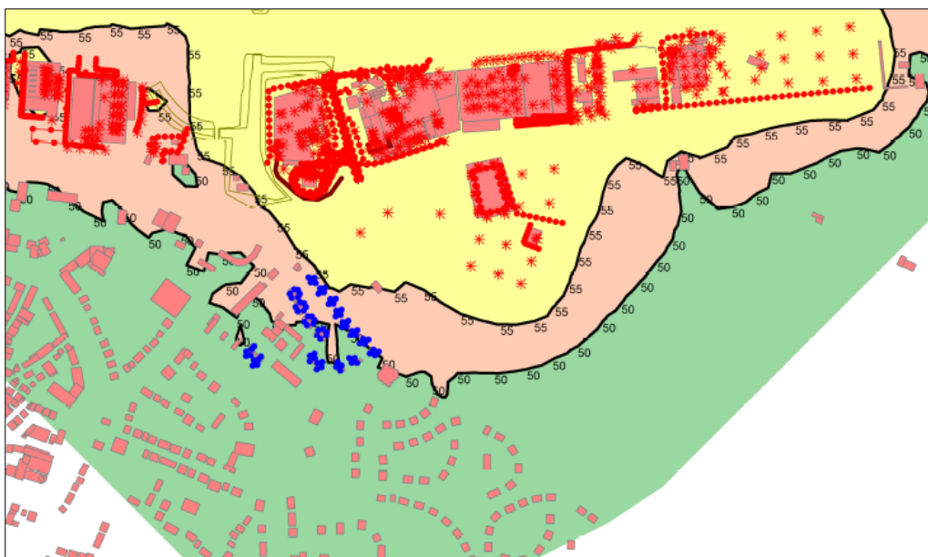
Figuur 2 Ligging geluidscontouren industrielawaai geluidsgezoneerde industrieterrein én bedrijventerrein Hanzeweg inclusief correcties, beoordelingshoogte 5 meter
