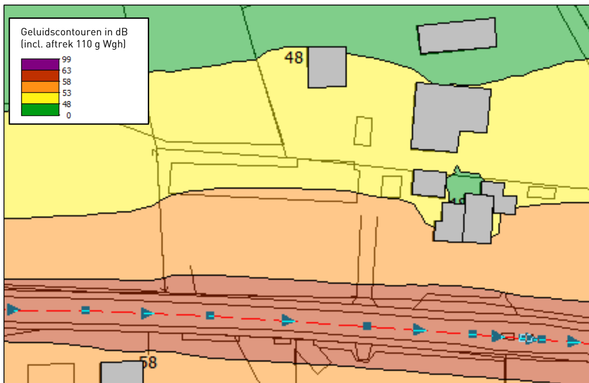
Figuur 6: Ligging van de geluidscontouren
