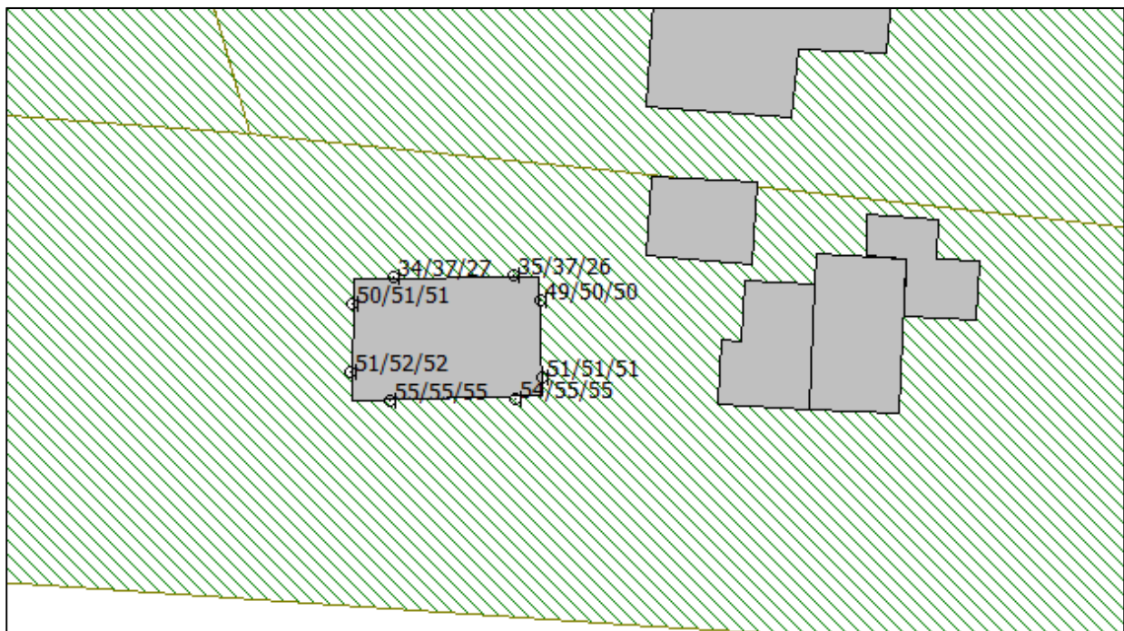
Figuur 7: Cumulatieve geluidsbelastingen ( L_{CUM,plus} )
