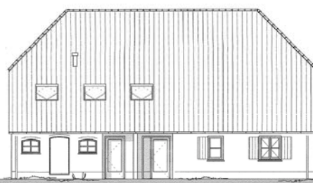
nieuwe L.Zijgevel
