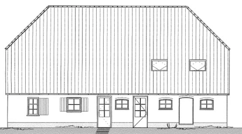
Nieuwe R.Zijgevel
