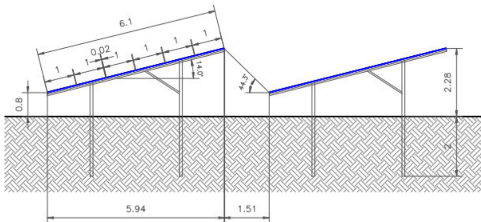
Afbeelding 9: Doorsnede van de basisconstructie
