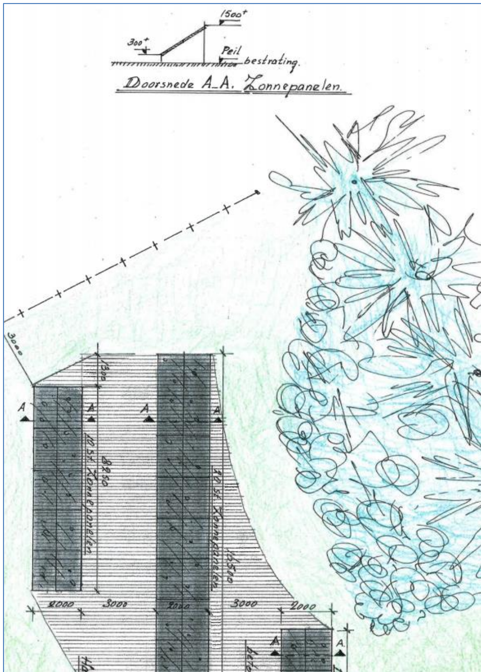
Figuur 7: Tekening dwarsdoorsnede zonnepanelen
