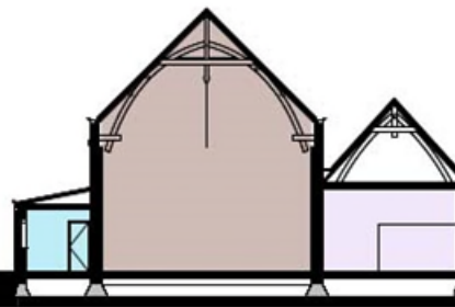
doorsnede B-B
