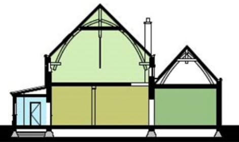
doorsnede C-C
