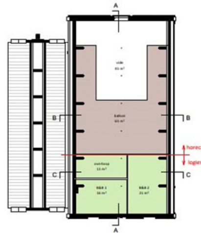
verdieping
