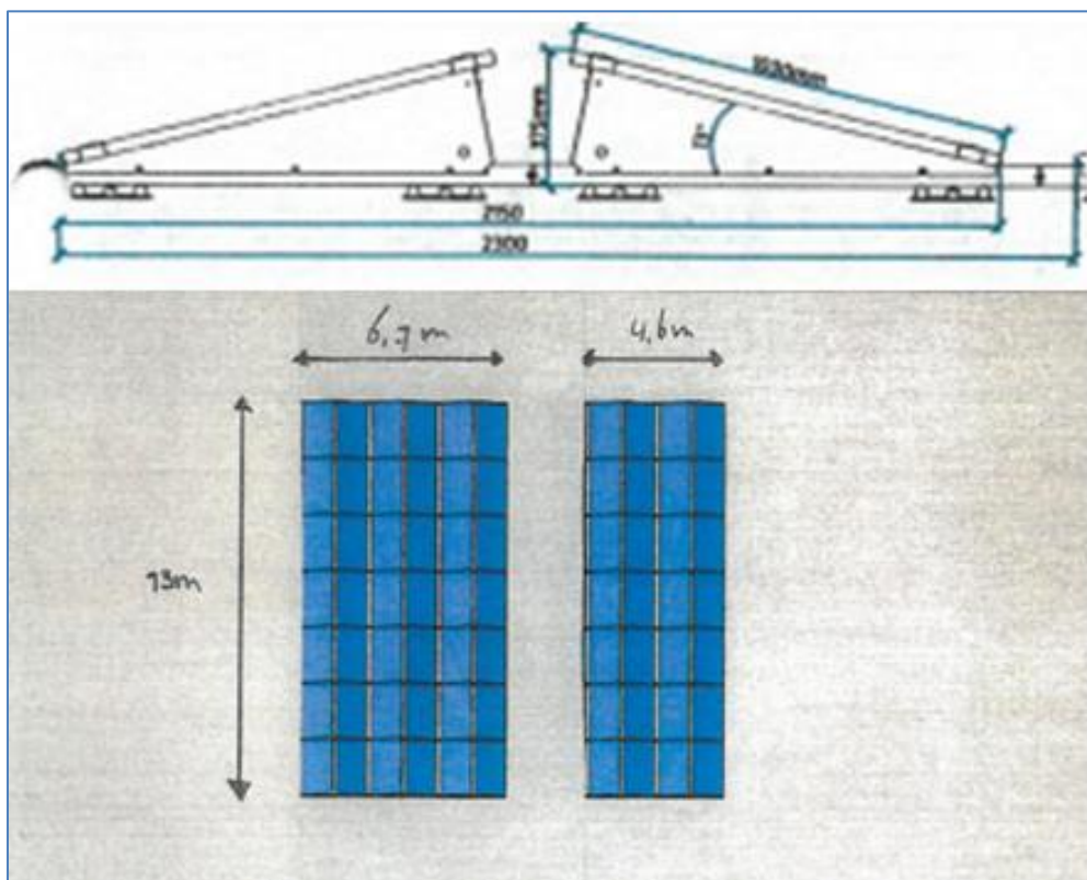
Figuur 6. Maatvoering (hoogte 0,4 meter) en doorsnede opstelling zonnepanelen
