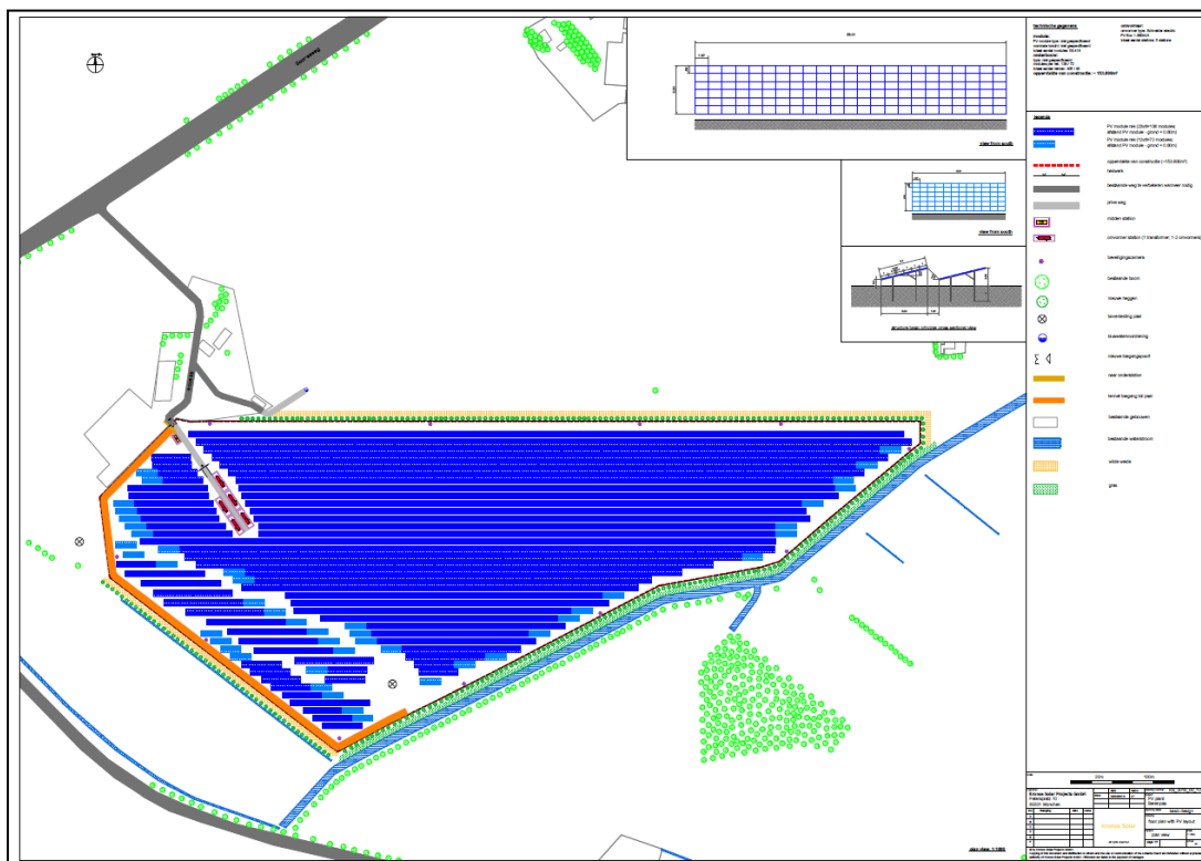
Figuur 7. Schets nieuwe situatie (bron: Kronos Solar Projects GmbH).
