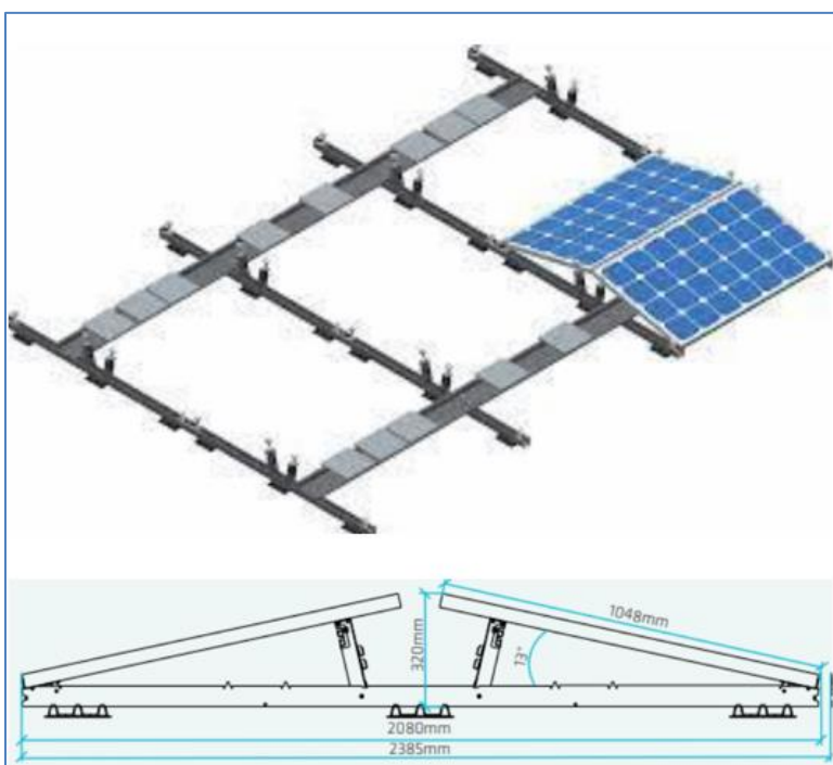
Afbeelding 5: Opbouw van de zonne-installatie
