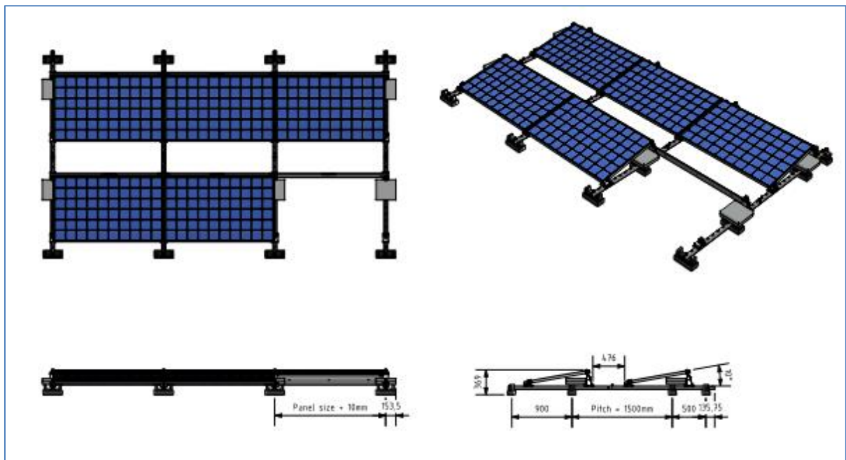
Figuur 6. Tekening van de zonne-installatie. De maximale hoogte bedraagt 0,4 meter.
