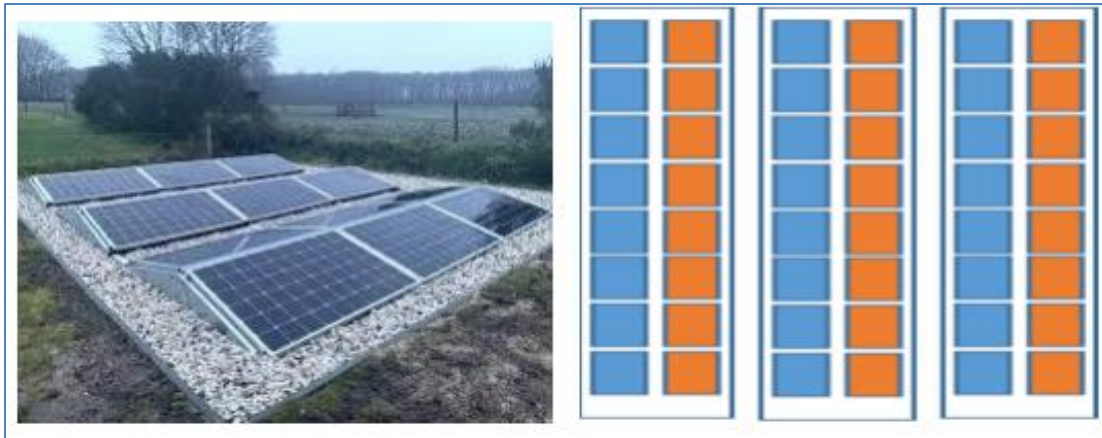
Afbeelding 5. Indicatie opstelling (blauw is westzijde; oranje is oostzijde)
