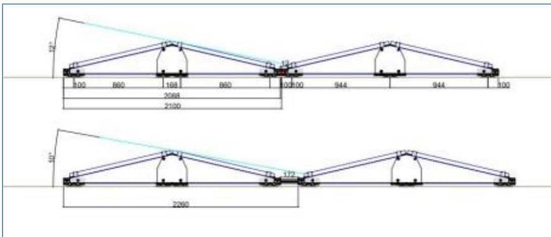
Afbeelding 6. Afmetingen van de opstelling. De maximale hoogte bedraagt 0,35 meter.
