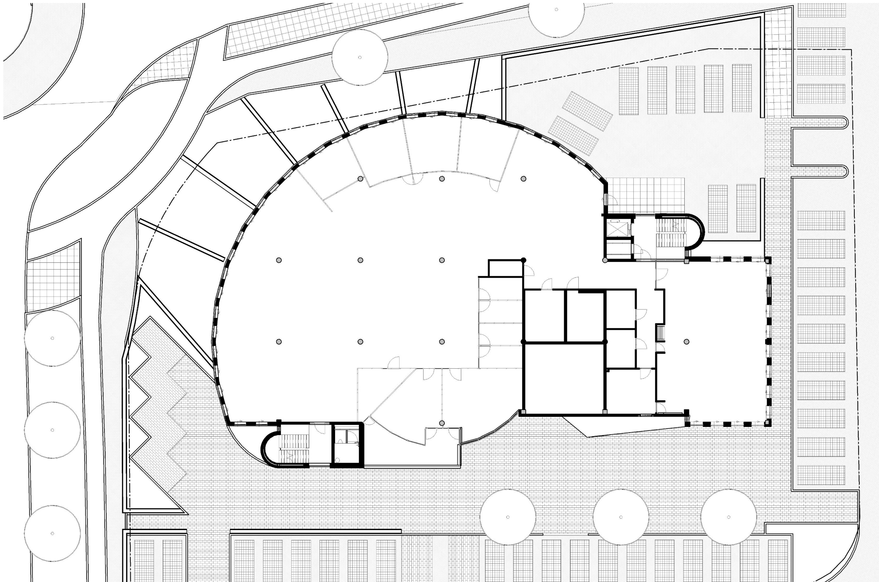
EERSTE VERDIEPING BESTAAND
