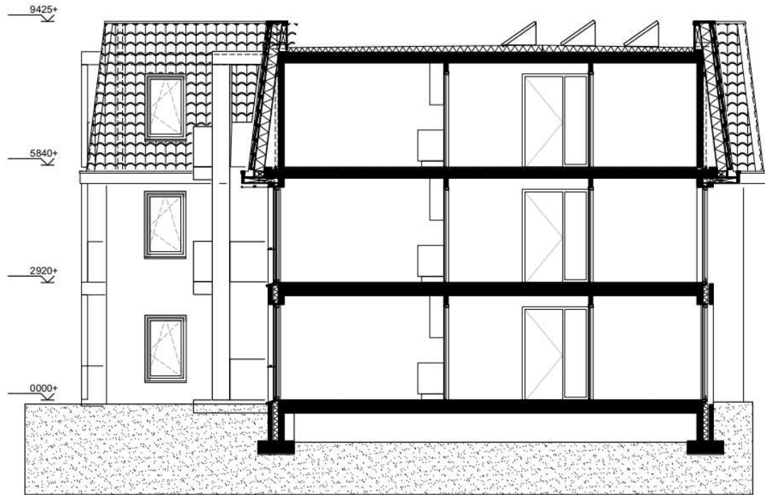
Afbeelding 7: Doorsnede (bron: Halma Architecten)
