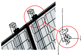
Detail eindklemmen
