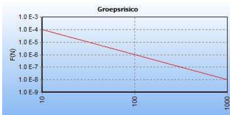
5.4 Figuur 5.4 FN curve voor 8530_leiding-N-576-77-deel-1 van N.V. Nederlandse Gasunie voor de kilometer tussen stationing 1290.00 en stationing 2030.00
