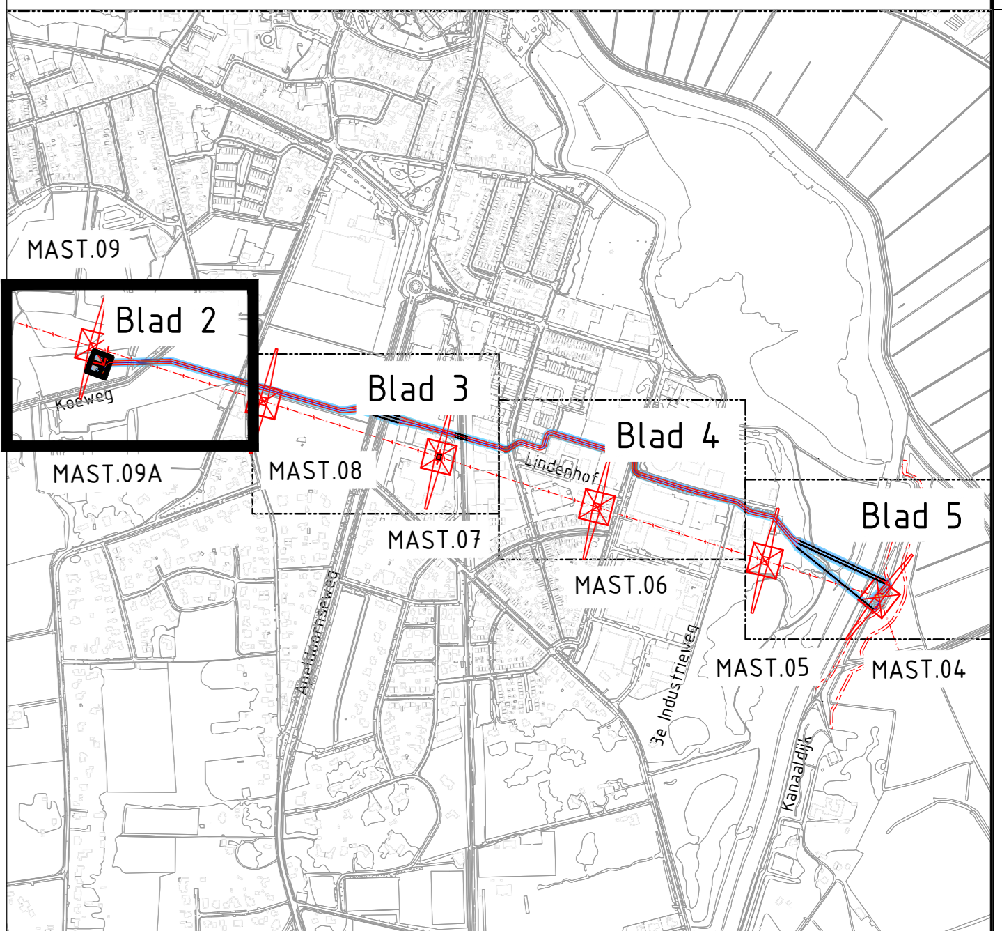
OVERZICHT SCHAAL 1 : 10000
