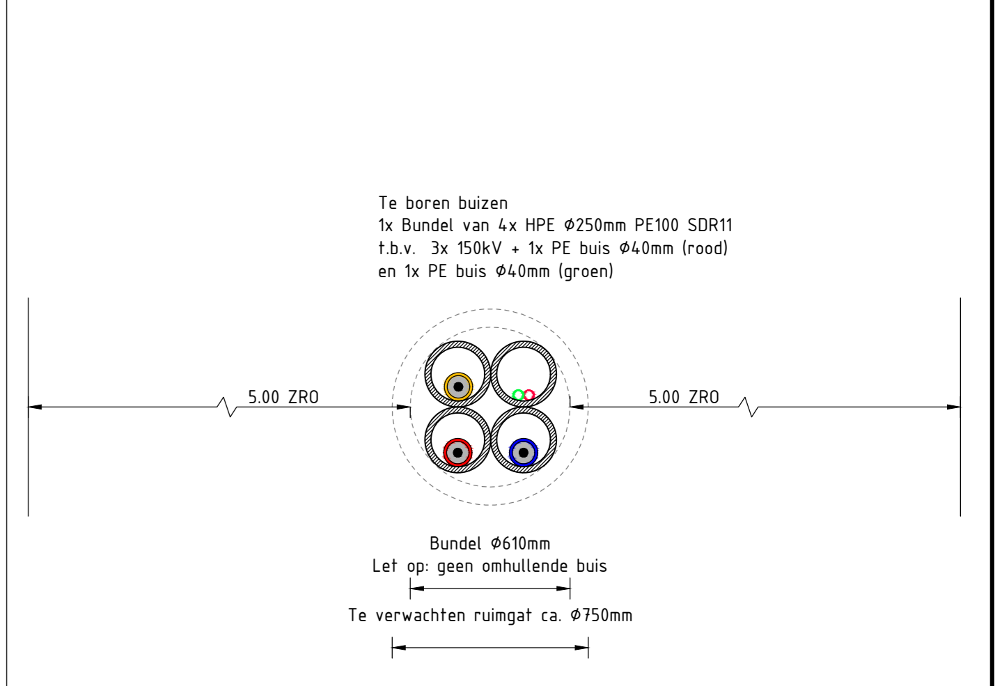
DWARSPROFIEL BORING C-C SCHAAL 1:20
