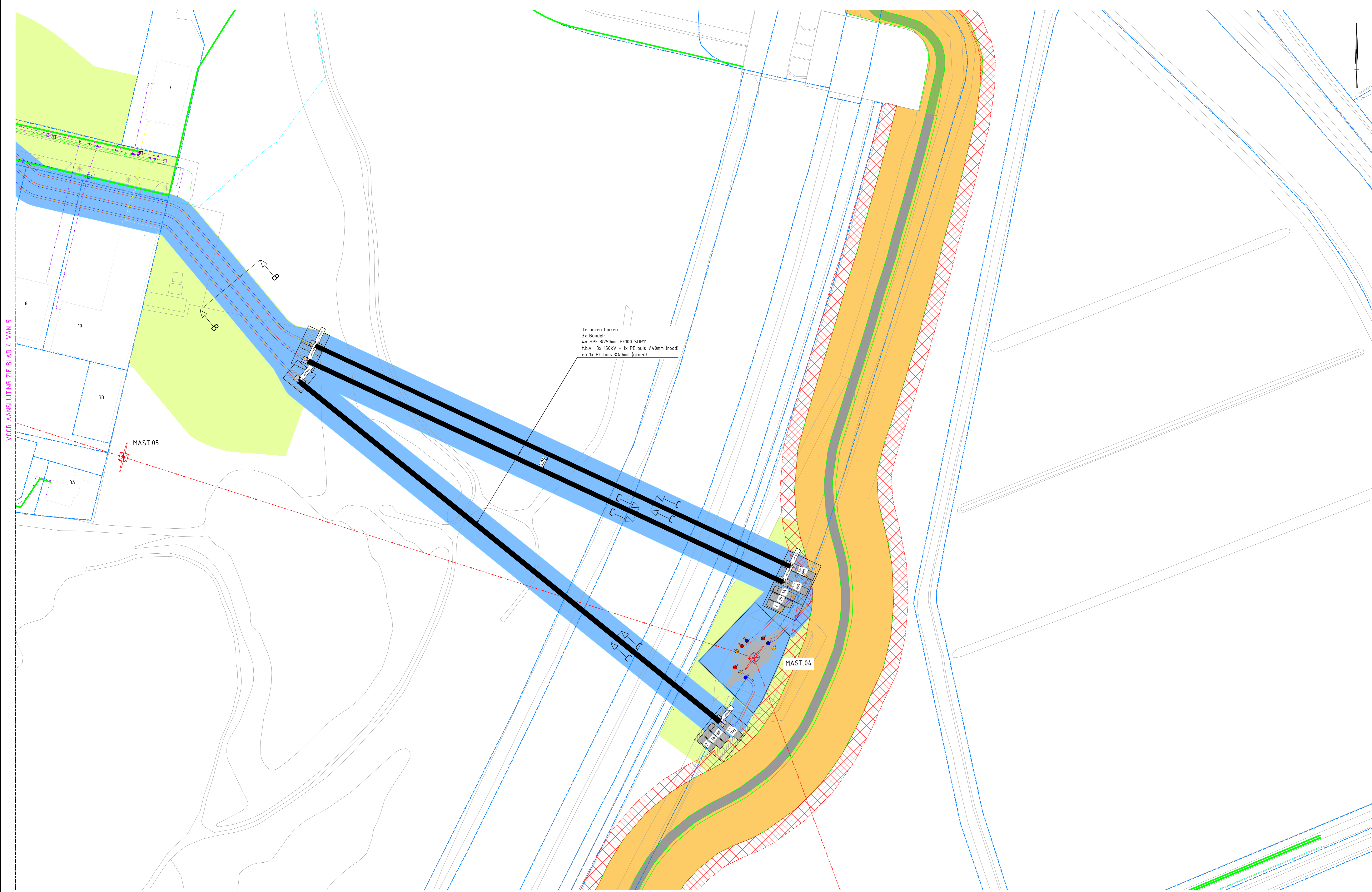
SITUATIE SCHAAL 1 : 500
