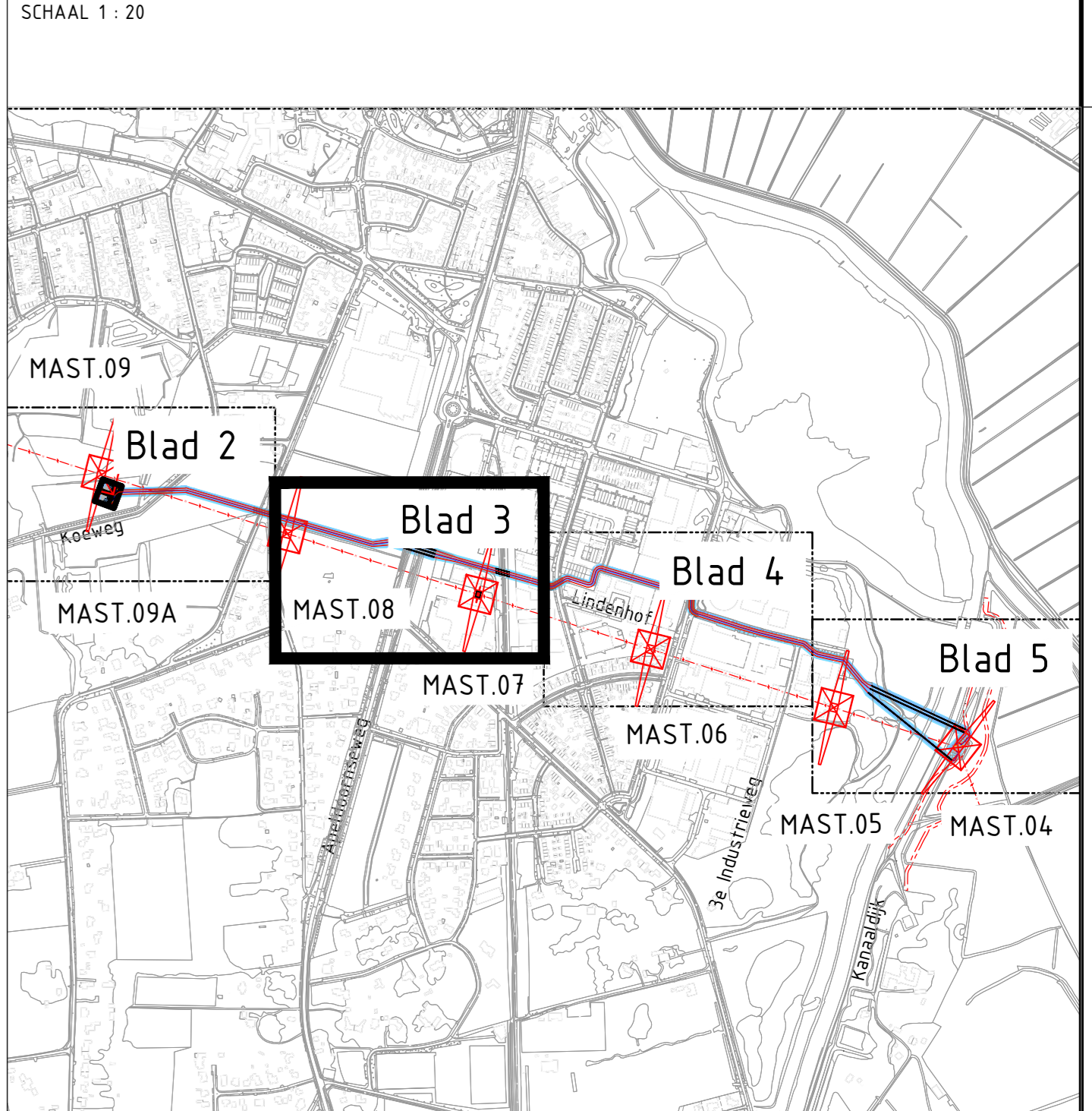
OVERZICHT SCHAAL 1:10000
