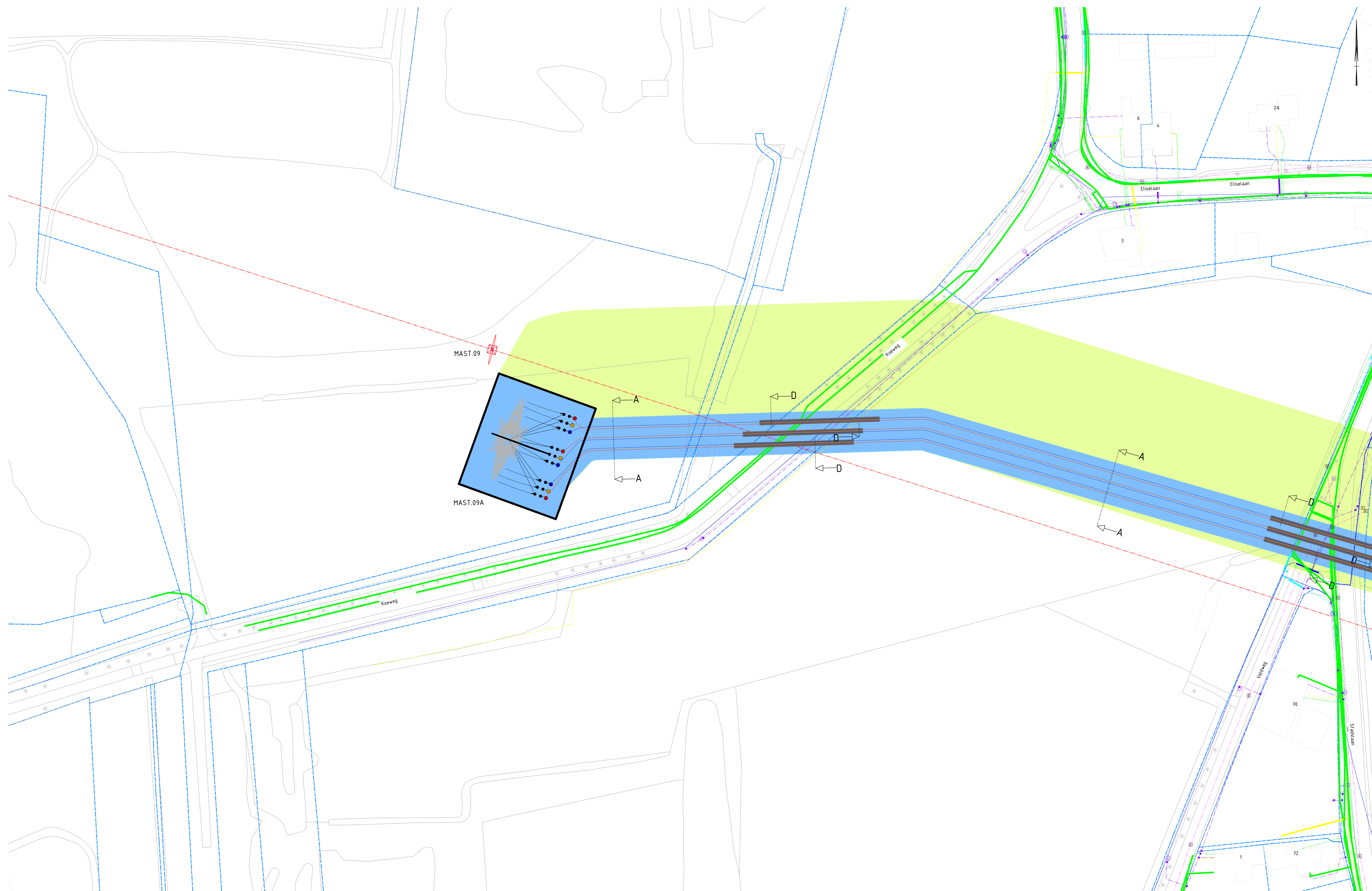
SITUATIE SCHAAL 1 : 500
