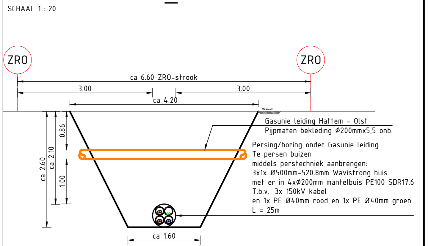
DWARSPROFIEL PERSING E-E SCHAAL 1:20
