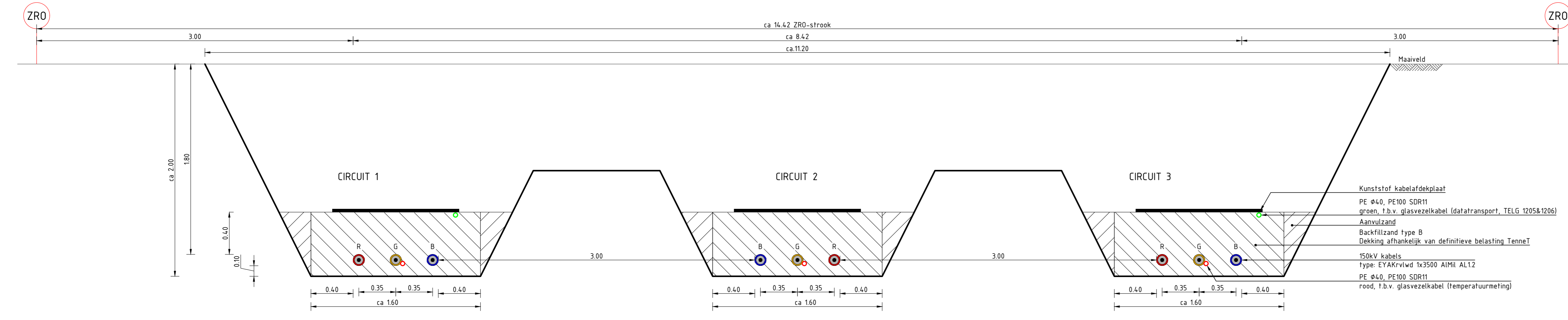
DWARSPROFIEL A-A_1.8 meter-MV SCHAAL 1 : 20
