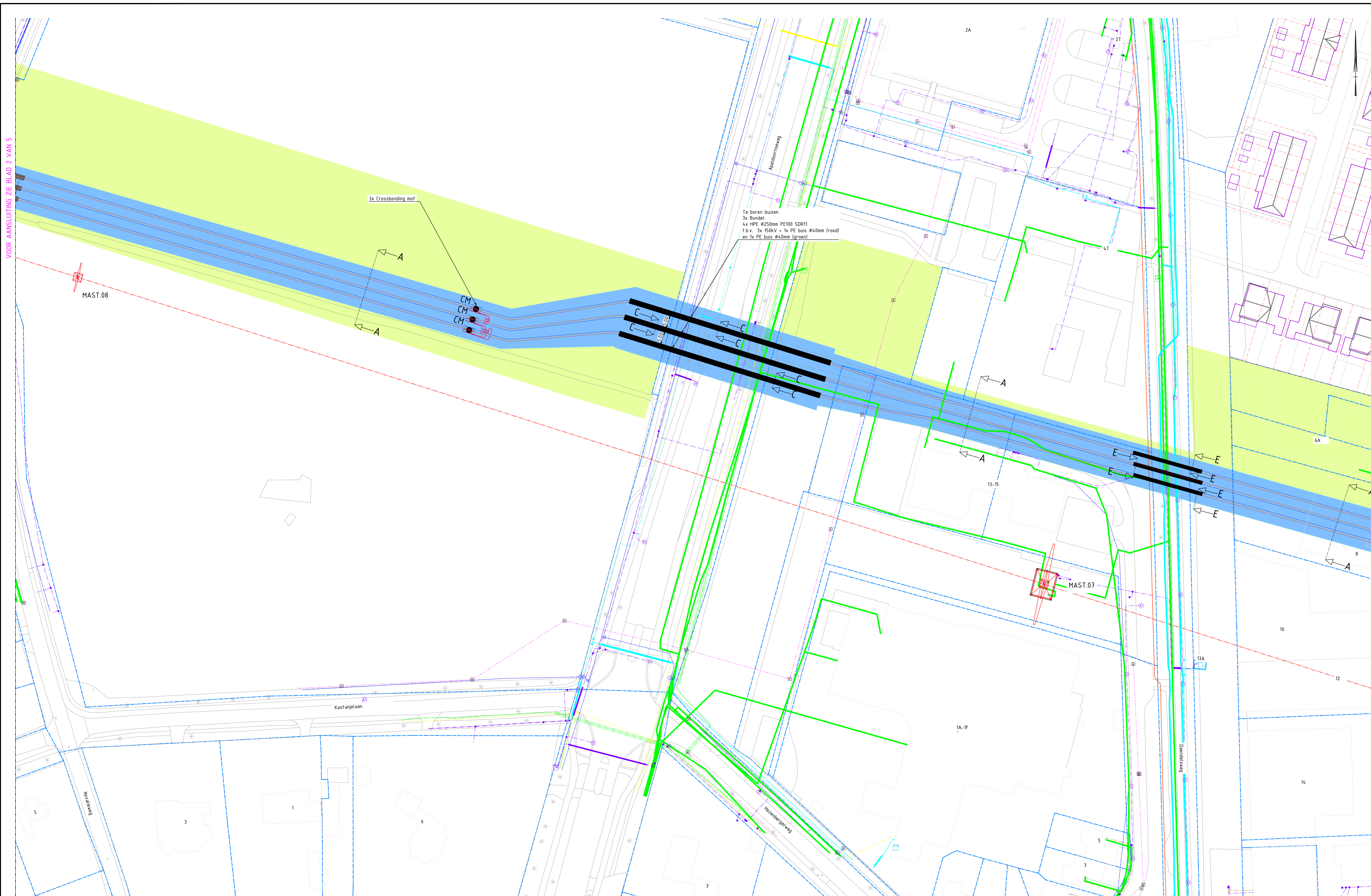
SITUATIE SCHAAL 1:500
