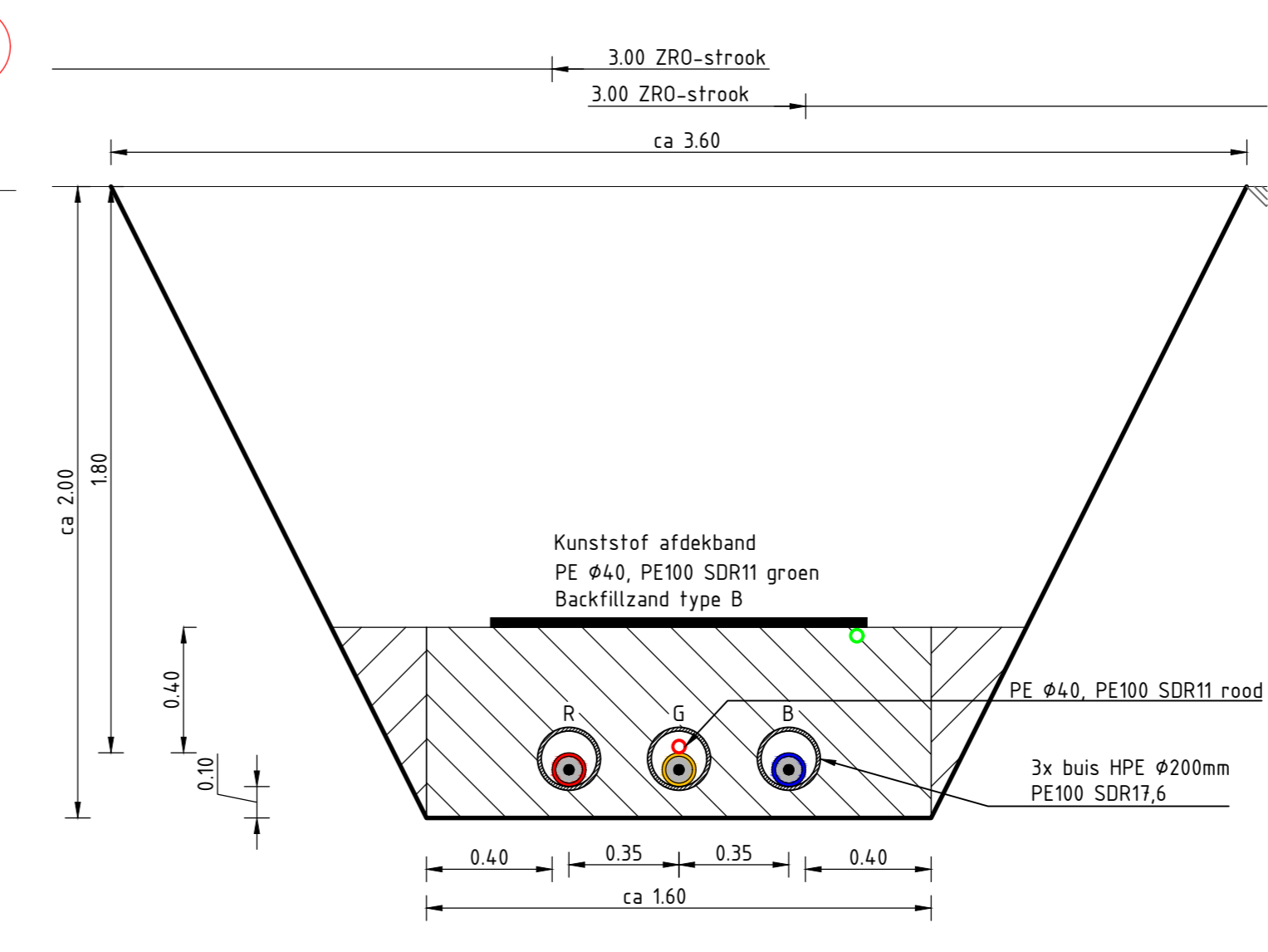
DWARSPROFIEL D-D SCHAAL 1 : 20
