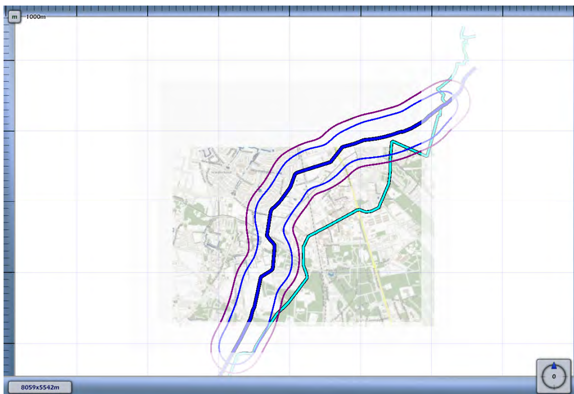
3.1 Figuur 3.1 Plaatsgebonden risico voor leiding-A-510-deel-1 van N.V. Nederlandse Gasunie
