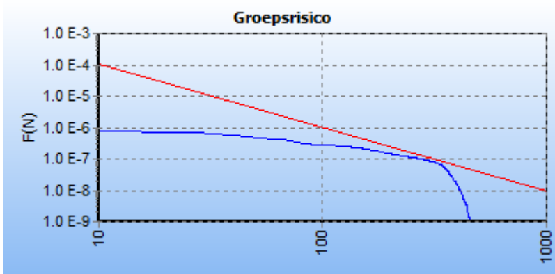
5.1 Figuur 5.1 FN curve voor leiding-A-510-deel-1 van N.V. Nederlandse Gasunie voor de kilometer tussen stationing 2040.00 en stationing 3040.00
