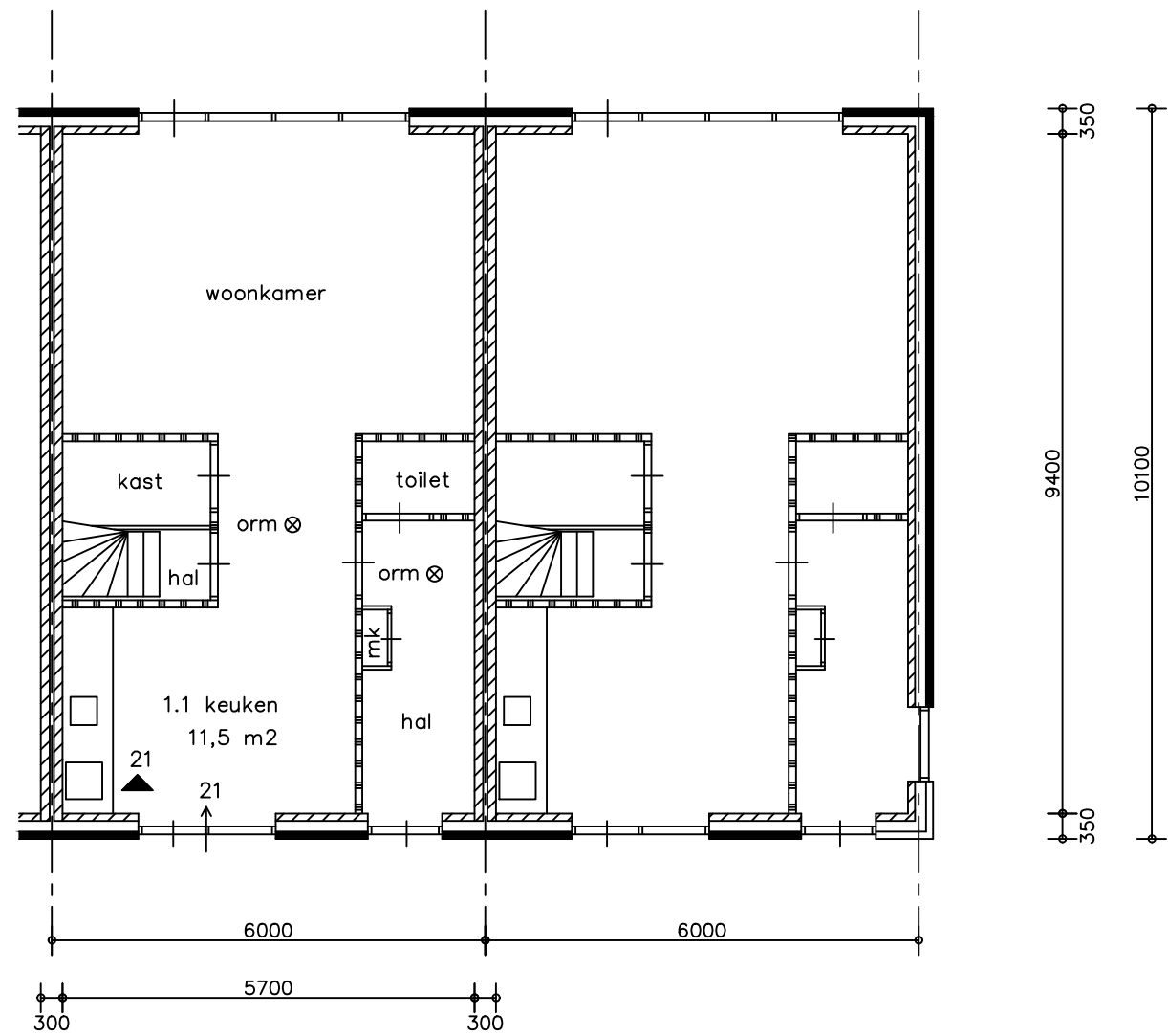
plattegrond bestaand
