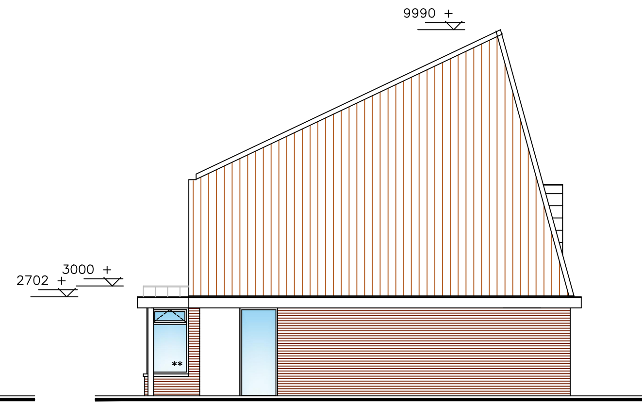
rechterzijgevel gewijzigd
