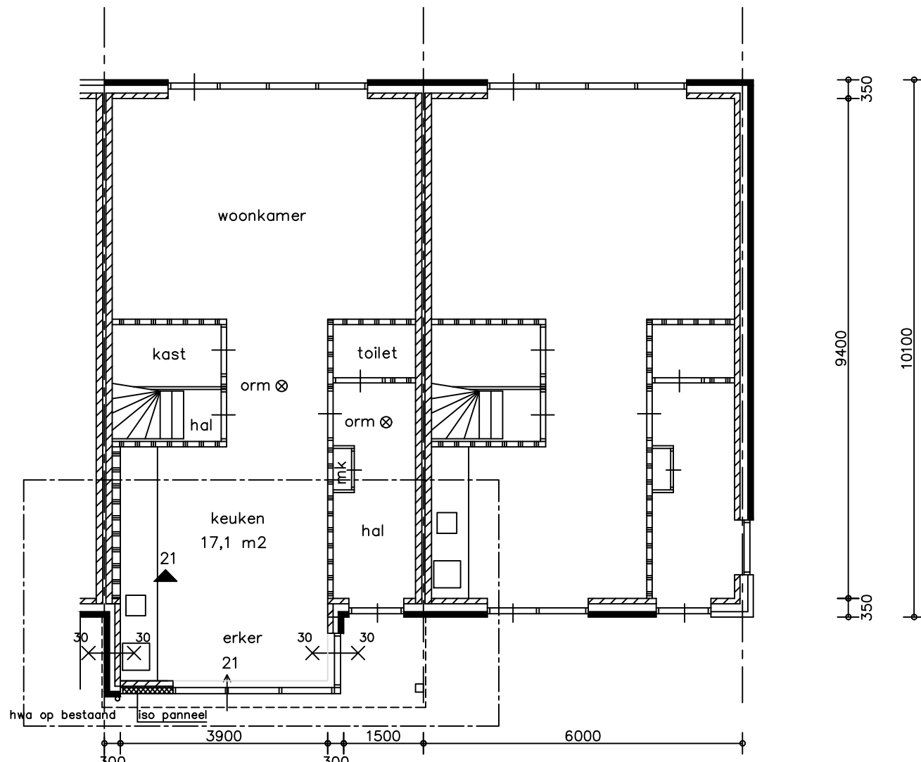
plattegrond gewijzigd
