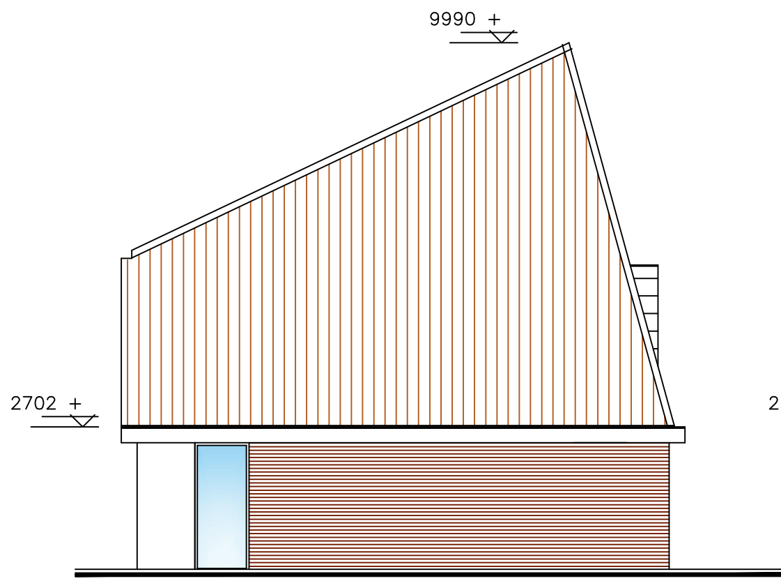
rechterzijgevel bestaand
