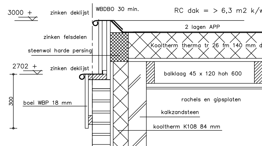
dakconstructie
