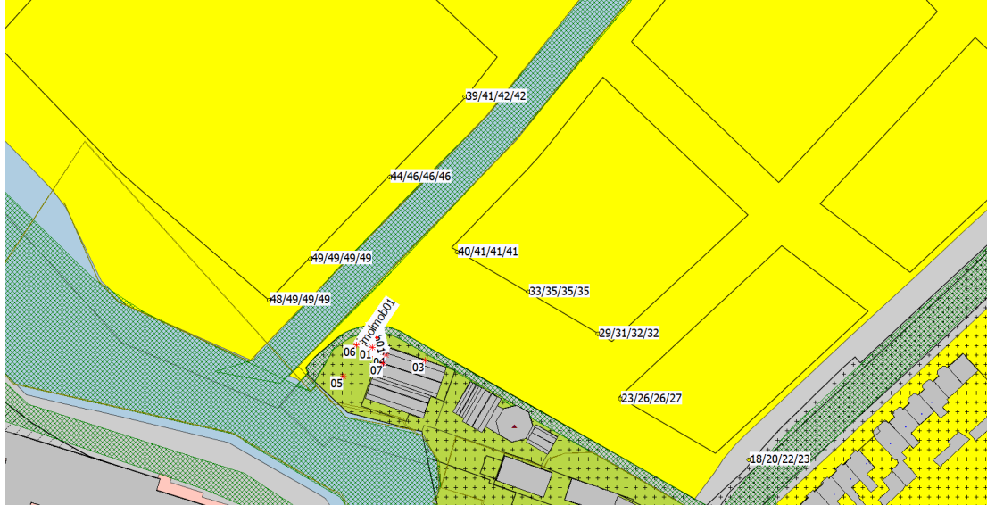
Figuur 4.1 L_{A,LT} Botterloods en de Vischafslag dagperiode (richtwaarde is 50 dB(A))
