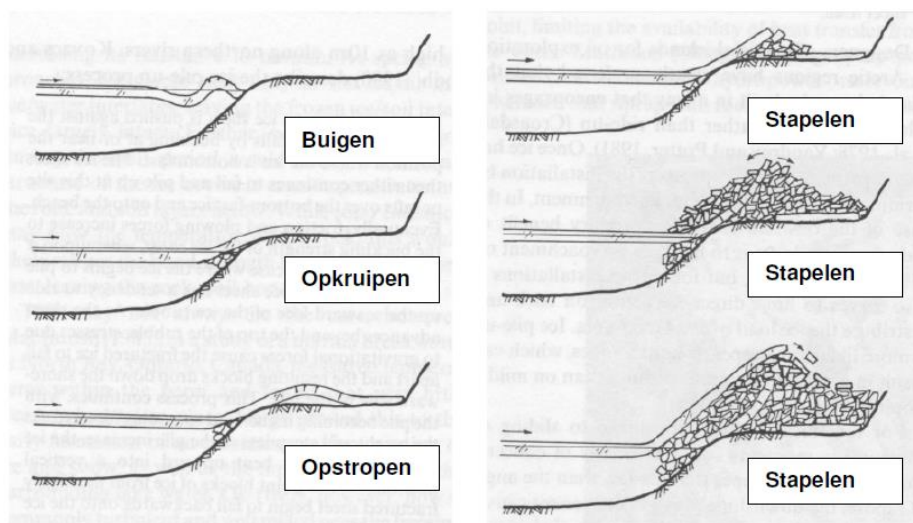
Figuur 26 Verschillende fasen in het opstapelen van kruiend ijs tegen een dijk.
