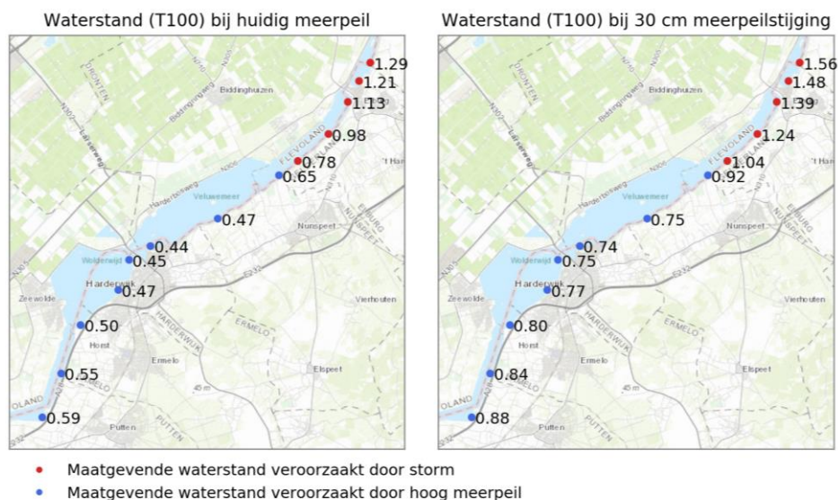
Figuur 6 Waterstanden in m+NAP bij het huidige meerpeil en bij een meerpeil- stijging met 30 cm. Het gaat om de waterstanden met een herhalings- tijd van 100 jaar.
