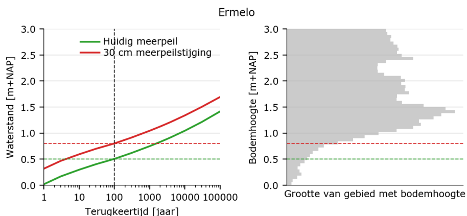
Figuur 16 Waterstands- frequenties en bodemhoogtes voor Ermelo
