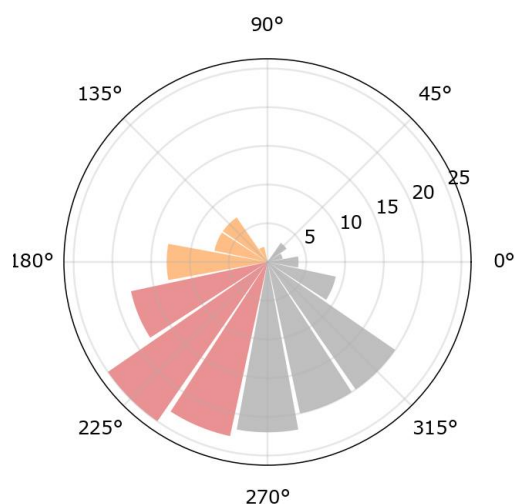
Figuur 25 Windrichtingen tijdens doorperiode na vorst. De grote van het 'blad' geeft het aantal gebeurtenissen in die richting weer.
