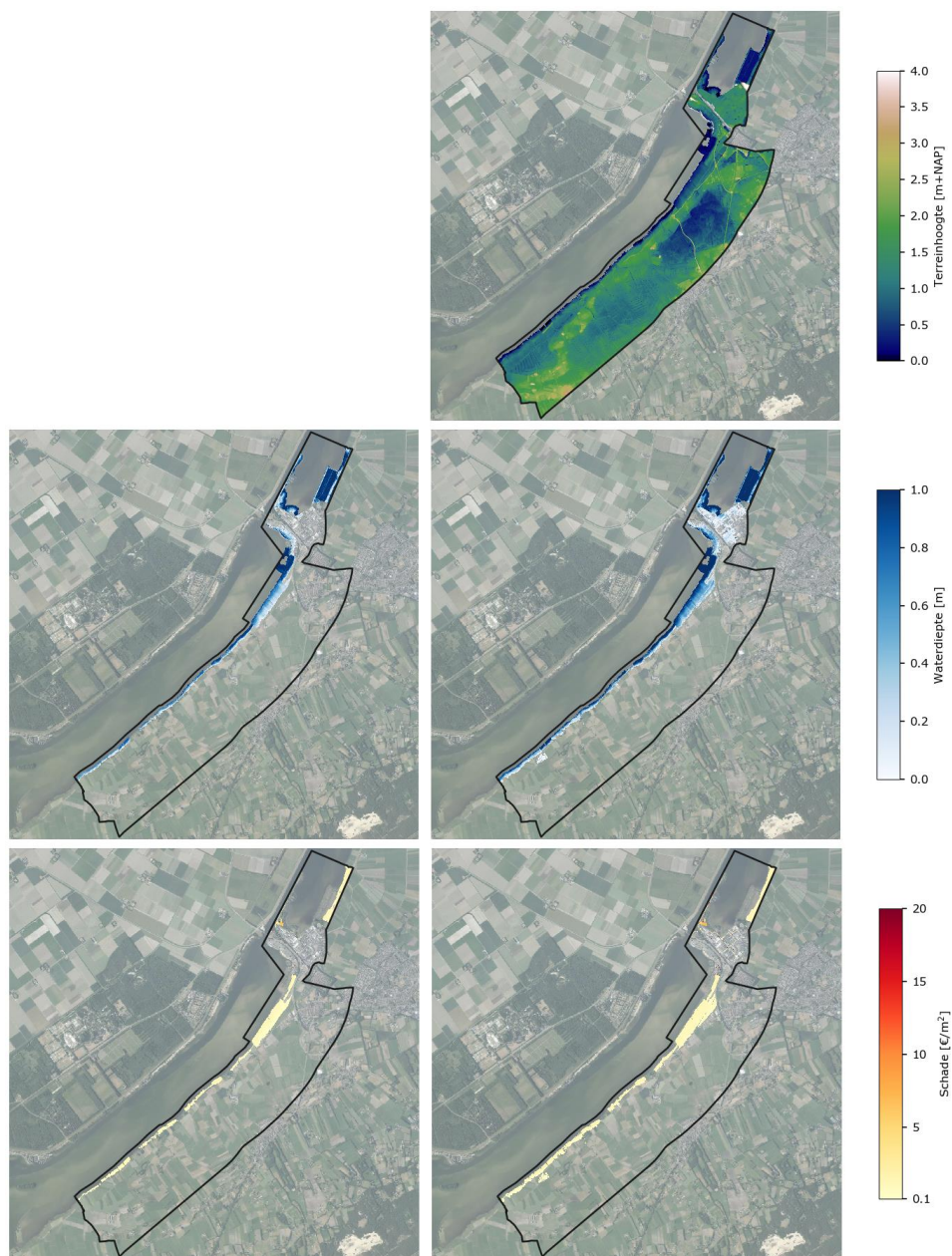
Figuur 21 Bodemhoogte, waterdiepte en schades voor Elburg bij een herhalingstijd van 100 jaar.
