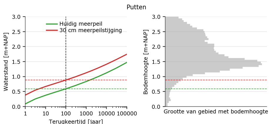
Figuur 13 Waterstands- frequenties en bodemhoogtes voor Putten
