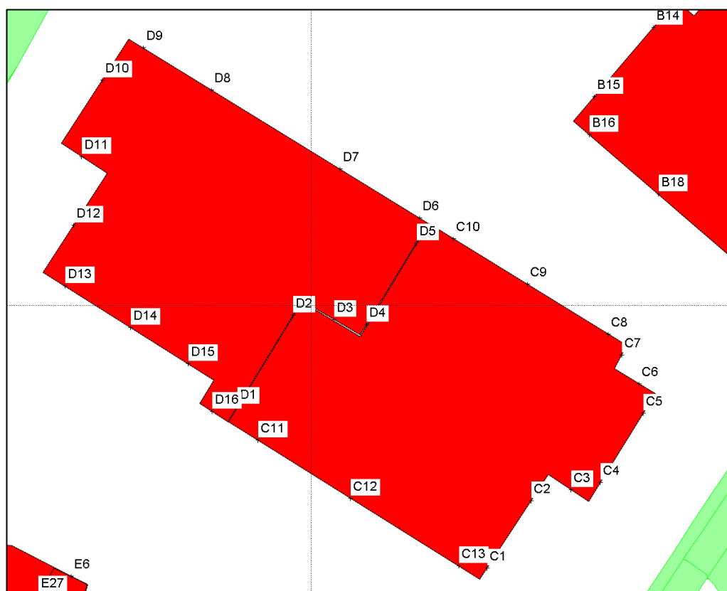
Figuur 4B Nummering waarneempunten gebouwen C en D, bewerking: SAB
