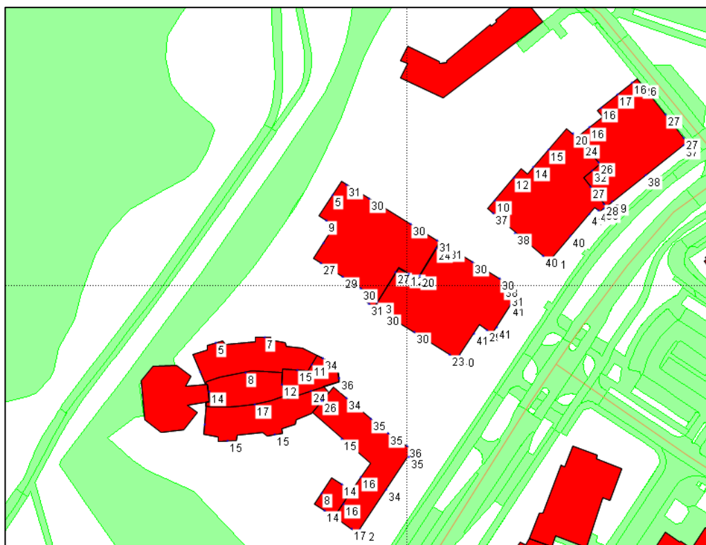
Figuur 10 Hoogst berekende geluidbelasting vanwege de Kruithuis (30 km/uur)
