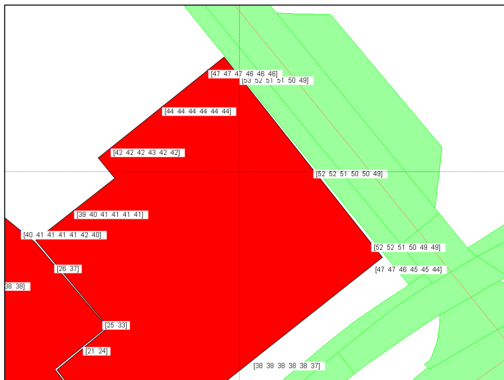
Figuur 9B Berekende geluidbelasting vanwege de Plantage (30 km/uur) per waarneemhoogte
