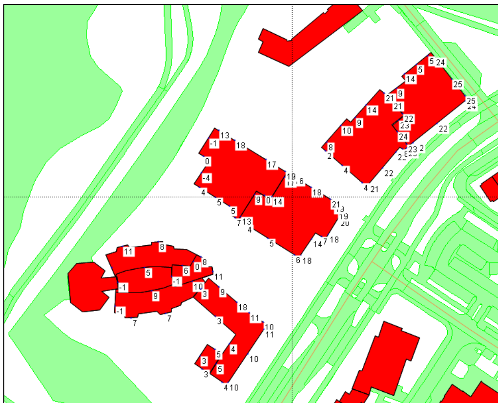
Figuur 7 Hoogst berekende geluidbelasting vanwege de Stationslaan (30 km/uur)
