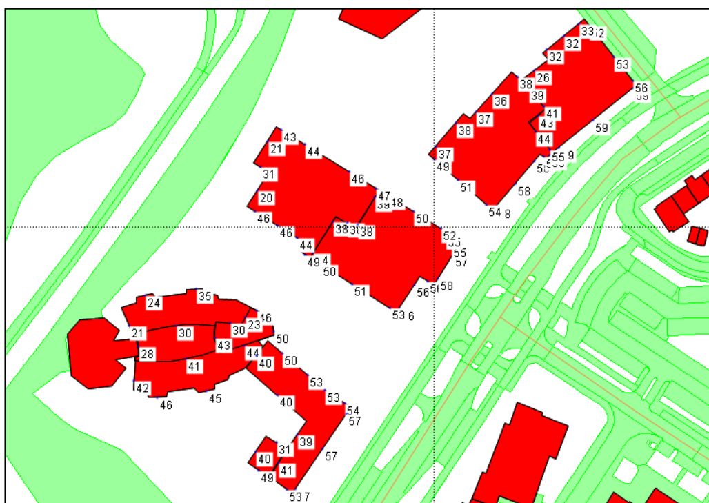
Figuur 5A Hoogst berekende geluidbelasting vanwege de Westeinde
