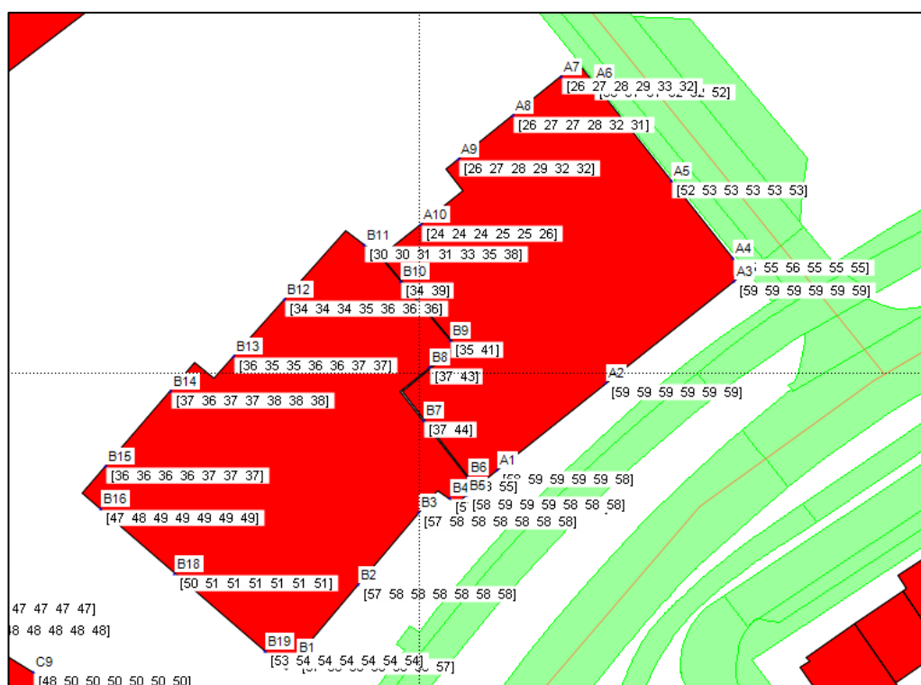
Figuur 5B Berekende geluidbelasting vanwege de Westeinde per waarneemhoogte
