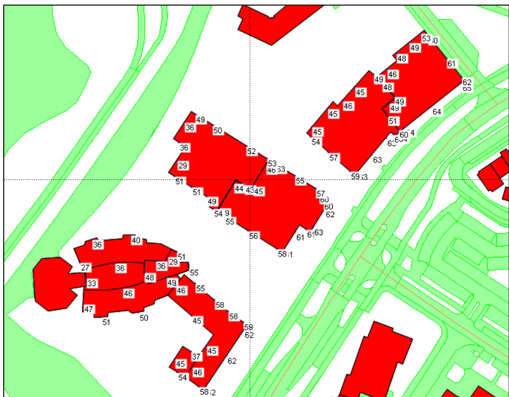
Figuur 11 Hoogst berekende gecumuleerde geluidbelasting exclusief aftrek art. 110g Wgh
