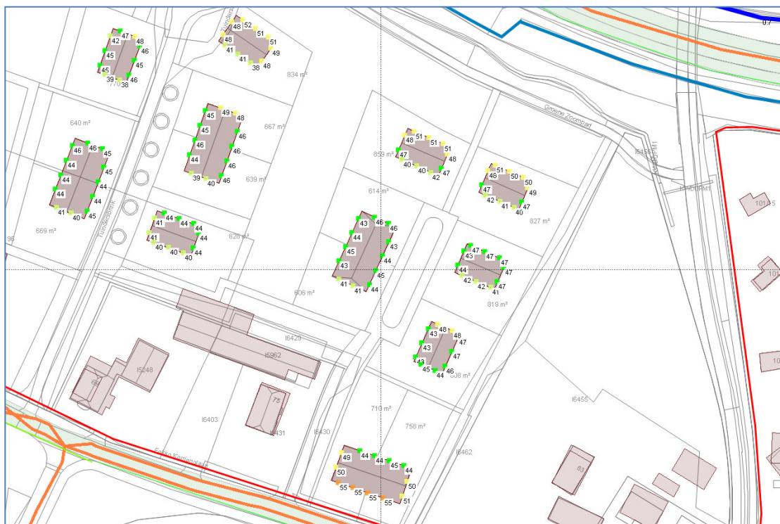
Figuur 7 Geluidbelasting ( L_{den} ) Fokko Kortlanglaan/ Horloseweg incl. aftrek stiller verkeer op woningen Tuindersbrink
