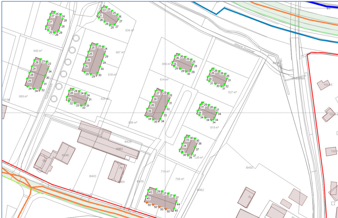
Figuur 7 Geluidbelasting ( L_{den} ) Fokko Kortlanglaan/ Horloseweg incl. aftrek stiller verkeer op woningen Tuindersbrink
