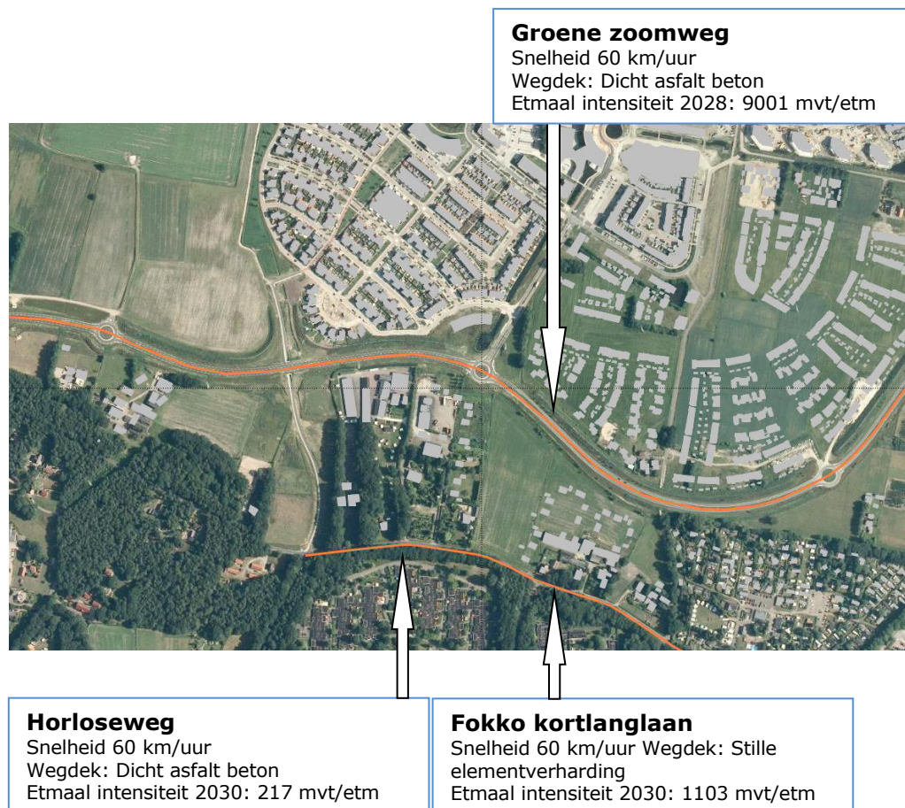
Figuur 4 Verkeersgegevens
