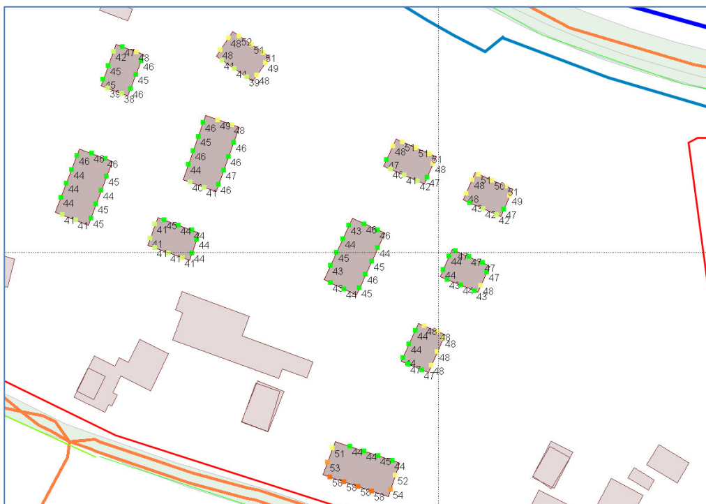
Figuur 8 Geluidbelasting Groene Zoomweg, Fokko Kortlanglaan/ Horloseweg gecumuleerd GES excl. aftrek stiller verkeer op woningen Tuindersbrink
