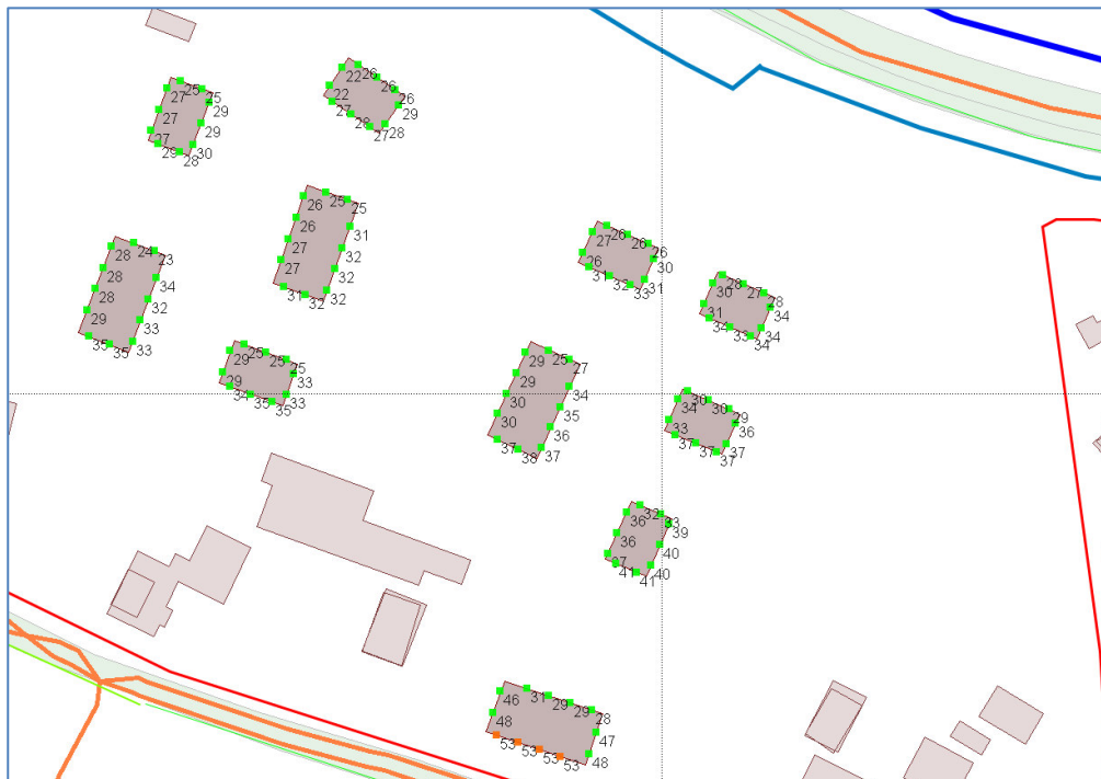
Figuur 7 Geluidbelasting ( L_{den} ) Fokko Kortlanglaan/ Horloseweg incl. aftrek stiller verkeer op woningen Tuindersbrink
