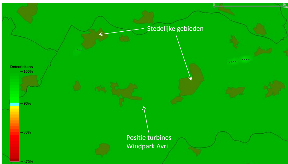
Figuur 5 Detectiekans van het MASS primaire verkeersleidingsradarnetwerk op 1000 voet boven het bouwplan voordat dit is gerealiseerd (baseline).
