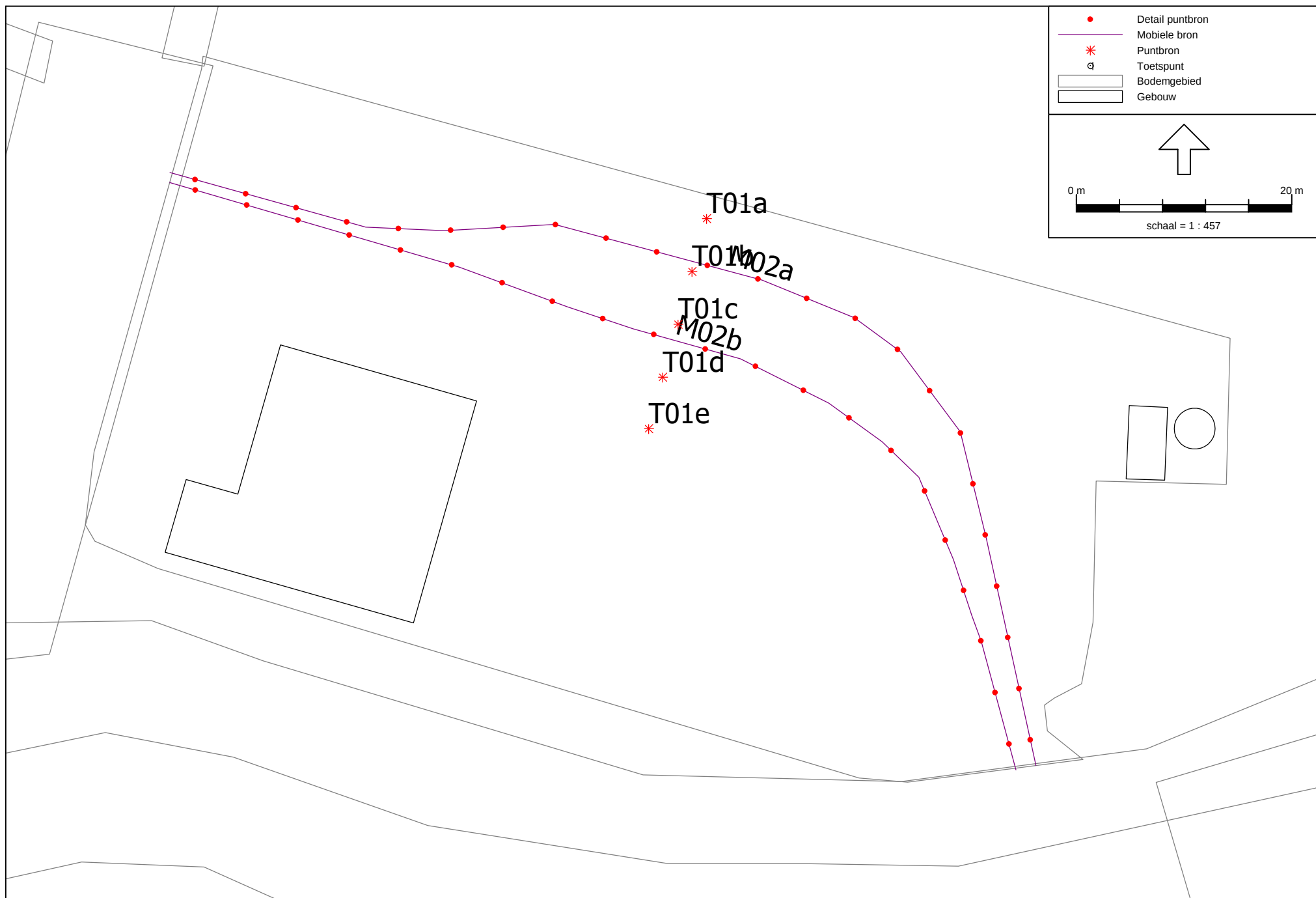
Figuur III-1-1 Overzicht geluidbronnen directe hinder vrachtauto's (tanken)
