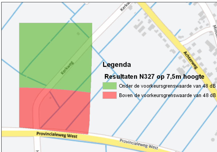
Figuur 3: resultaten N327 op 7,5 meter hoogte, 48 dB contour op ca. 155 m van wegas.
